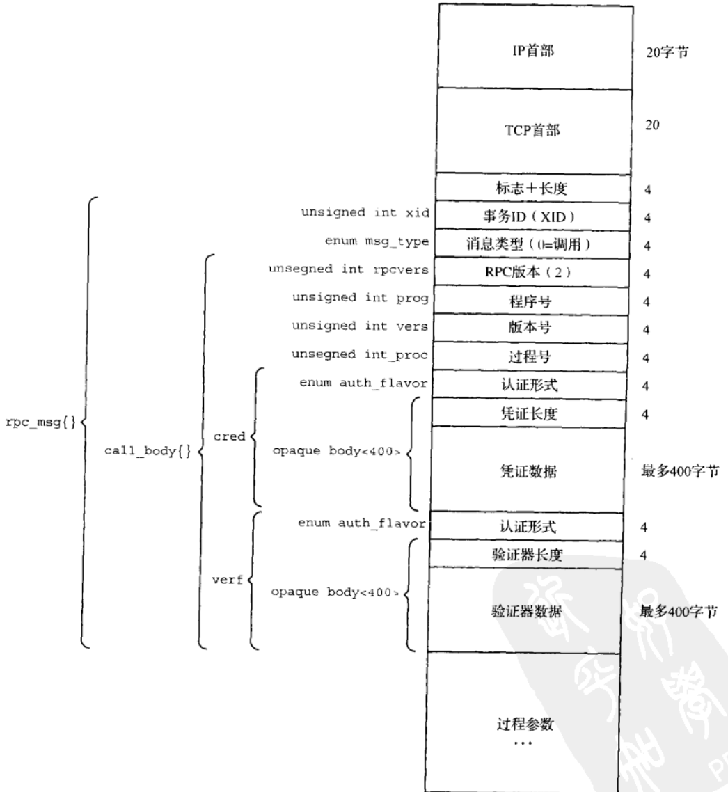
图16-30 封装在一个TCP分节中的RPC请求
