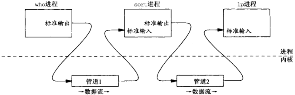
图4-5 某个shell管道线中三个进程间的管道
