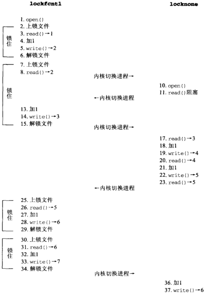
图9-6 loopfcntl和loopnone程序的时间线图
