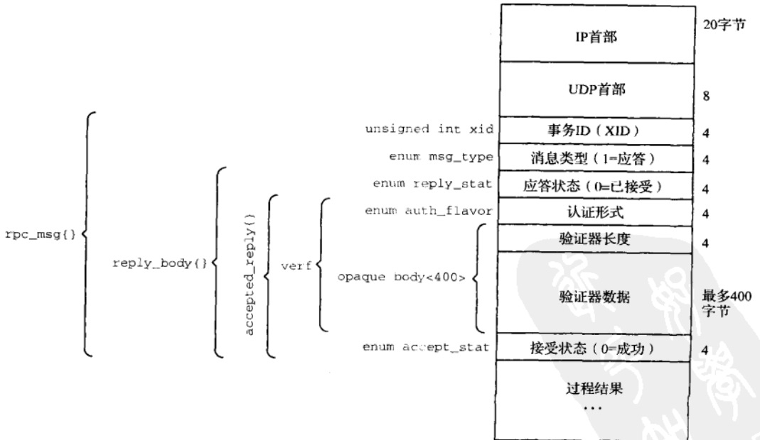
图16-32 封装为一个UDP数据报的成功的RPC应答
