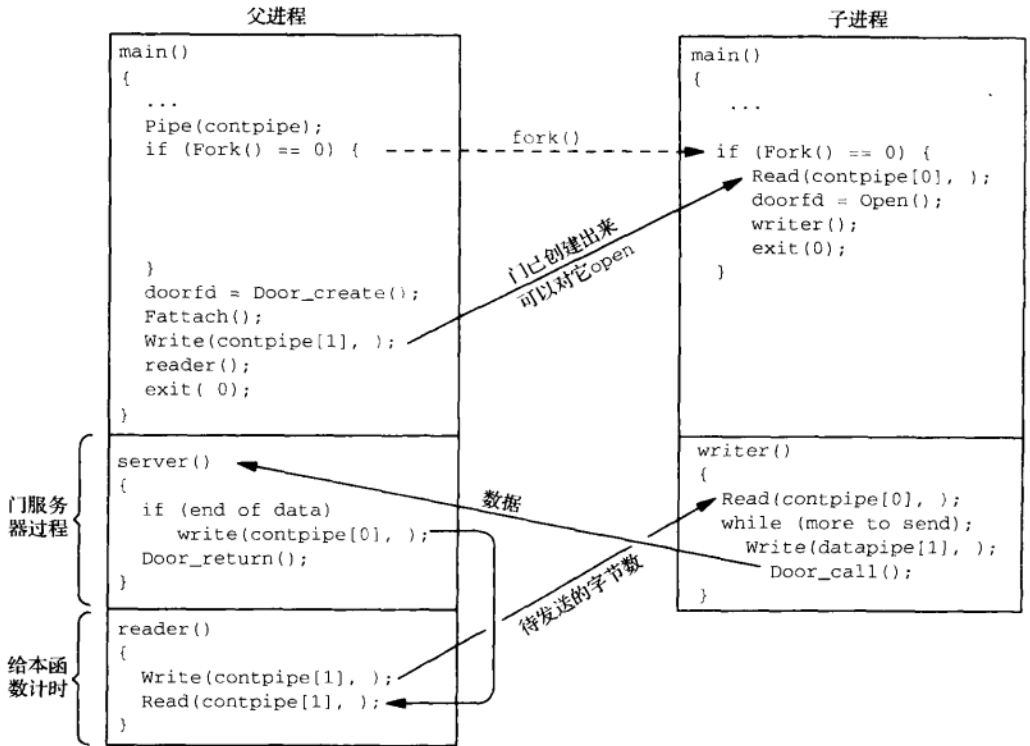
图A-23 门API带宽测量程序的概貌
