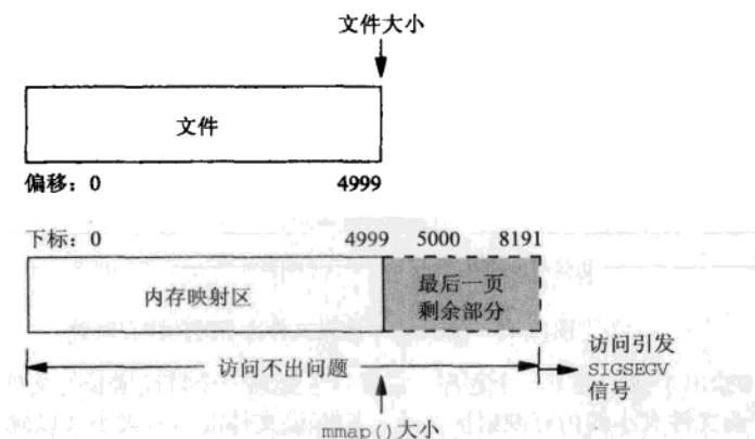
图12-17 mmap大小等于文件大小时的内存映射
