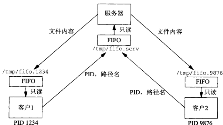
图4-22 单个服务器，多个客户
