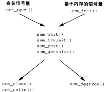
图10-6 用于Posix信号量的函数调用
