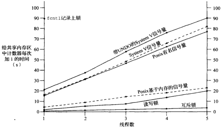
图A-7 给处于共享内存区中的一个计数器持续加1所需的时间 (Solaris 2.6)
