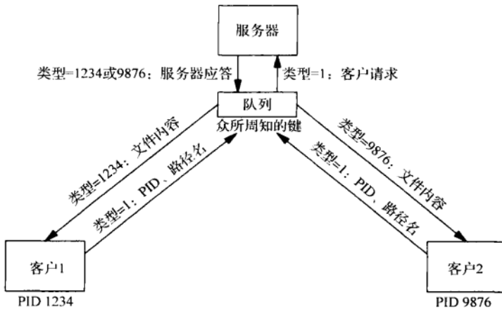
图6-14 在多个客户和单个服务器之间复用消息
