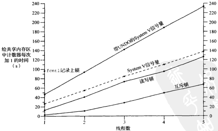
图A-9 给处于共享内存区中的一个计数器持续加1所需的时间 (Digital Unix 4.0B)
