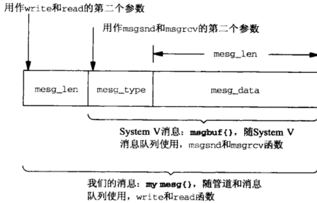
图4-26 我们的mymsg结构
