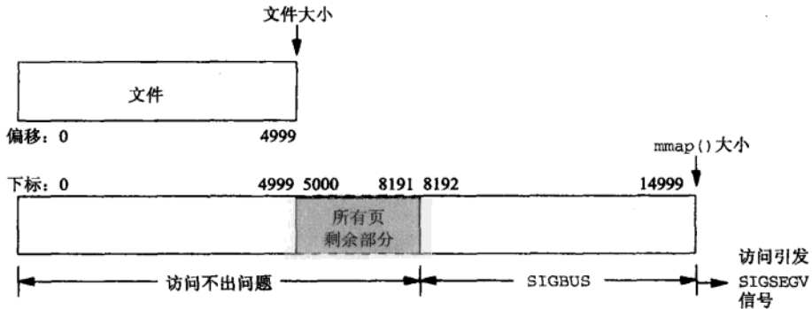
图12-18 mmap大小超过文件大小时的内存映射
