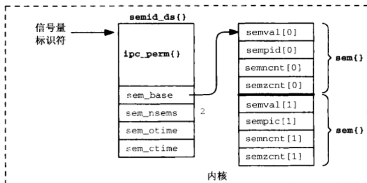
图11-1 由两组值构成的某个信号量集的内核数据结构
