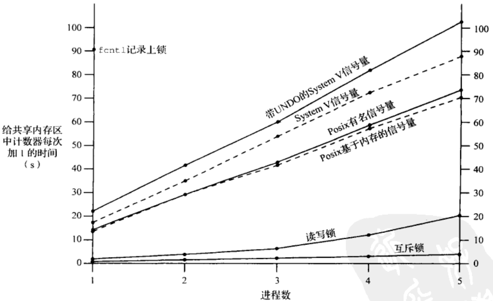
图A-11 给处于共享内存区中的一个计数器持续加1所需的时间 (Solaris 2.6)
