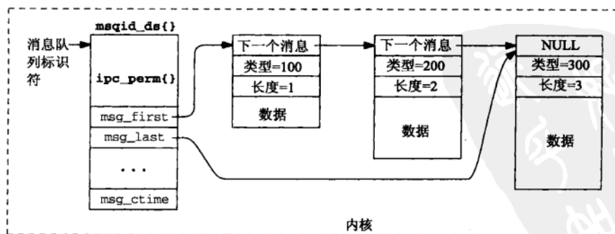
图6-1 内核中的System V消息队列结构
