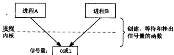
图10-1 由两个进程使用的一个二值信号量
