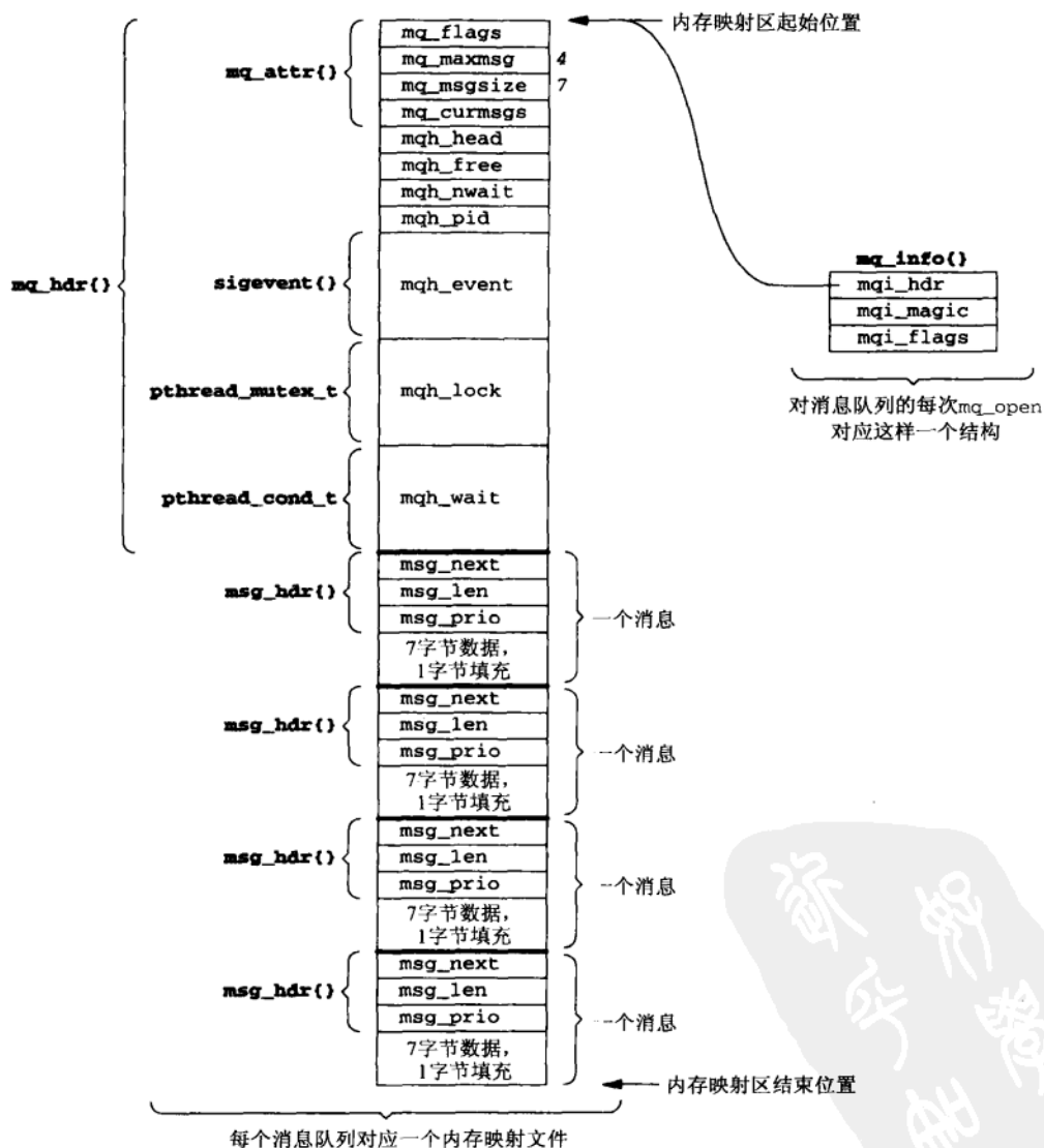
图 5-19 使用内存映射文件实现 Posix 消息队列的各种数据结构的布局
