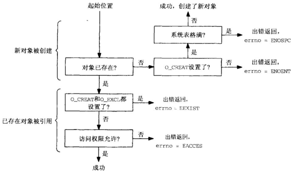
图2-5 打开或创建一个IPC对象的逻辑
