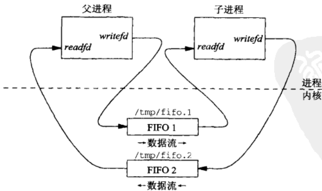
图4-17 使用两个FIFO的客户-服务器例子
