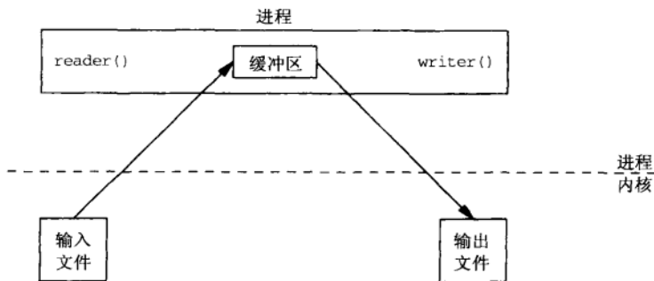
图10-27 由一个进程把数据读入某个缓冲区，再从该缓冲区写出
