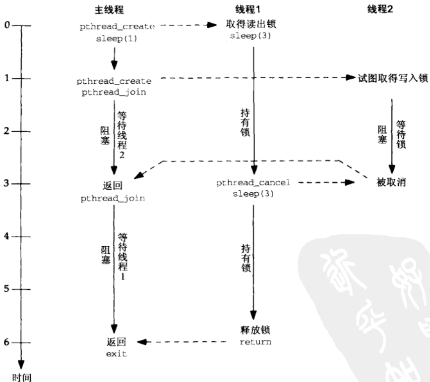
图8-9 图8-10中程序的时间线图
