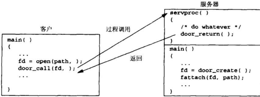
图15-4 从一个进程到另一个进程的表面过程调用
