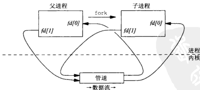
图4-3 单个进程内的管道，刚刚fork后
