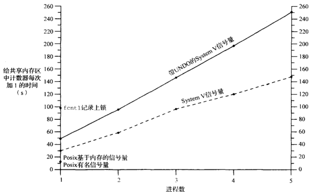
图A-13 给处于共享内存区中的一个计数器持续加1所需的时间 (Digital Unix 4.0B)
