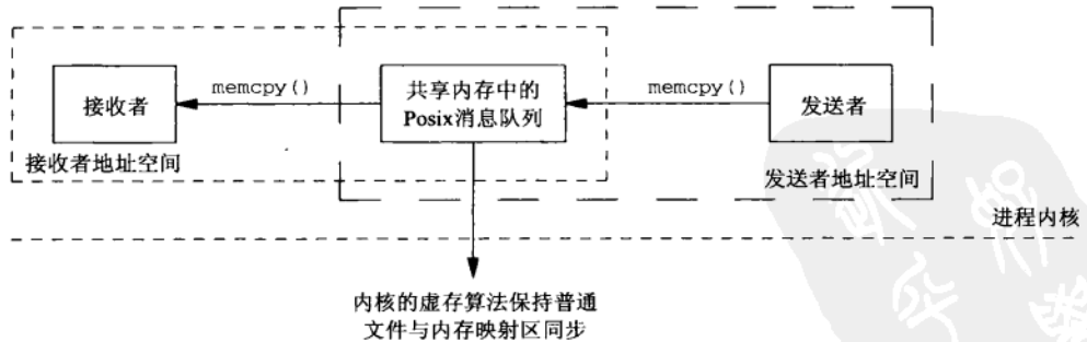
图D-8 使用通过mmap实现的Posix消息队列发送消息
