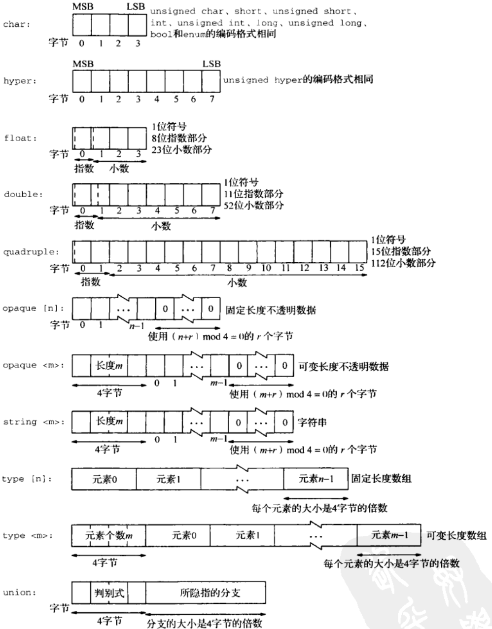
图16-15 XDR给它的各种数据类型采用的编码格式
