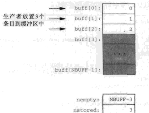
图10-15 生产者放置3个条目到缓冲区后的缓冲区和计数信号量
