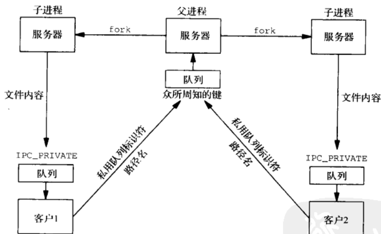
图6-19 每个服务器一个队列，每个客户一个队列
