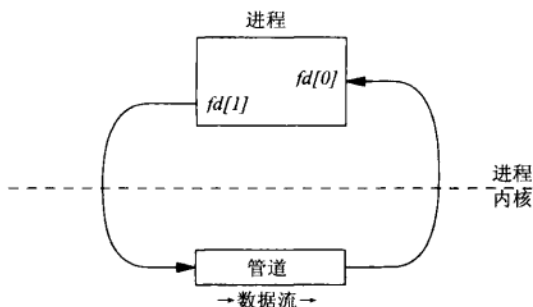
图4-2 单个进程中的管道
