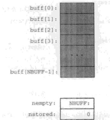
图10-14 初始化后的缓冲区和两个计数信号量
