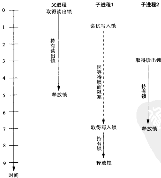
图9-7 确定有一个写入锁待处理期间是否允许有另一个读出锁
