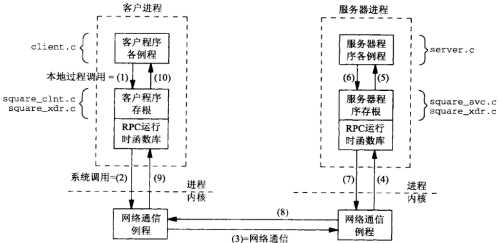
图16-5 一次远程过程调用中涉及的步骤
