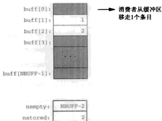
图10-16 消费者从缓冲区移走第一个条目后的缓冲区和计数信号量
