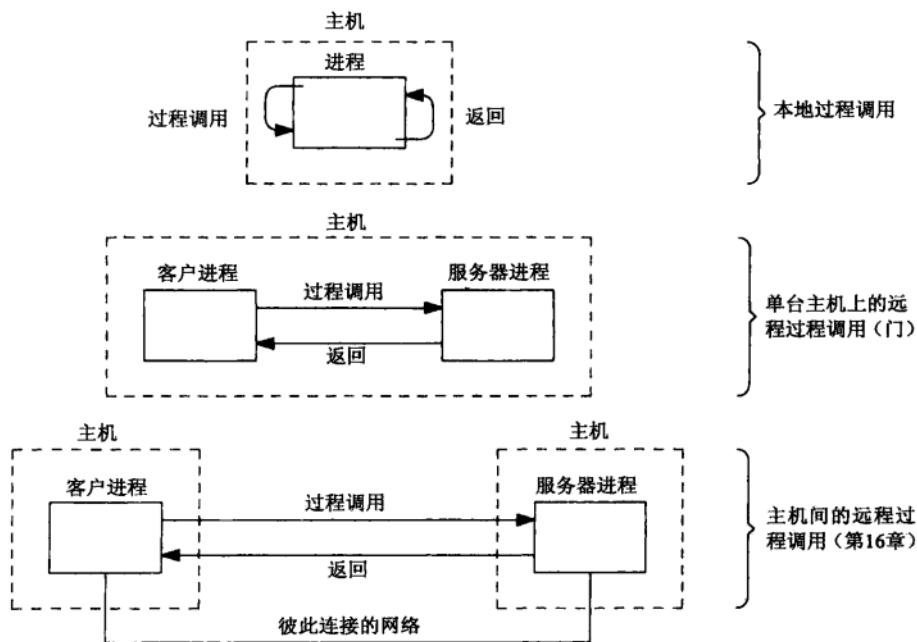
图15-1 三种不同类型的过程调用
