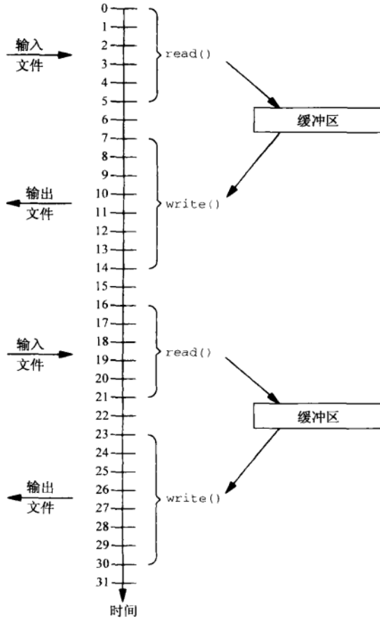
图10-28 由一个进程把数据读入某个缓冲区，再从该缓冲区写出
