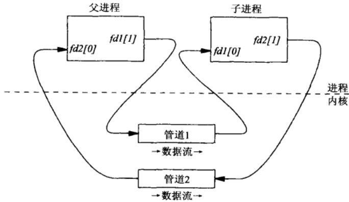
图4-6 提供一个双向数据流的两个管道
