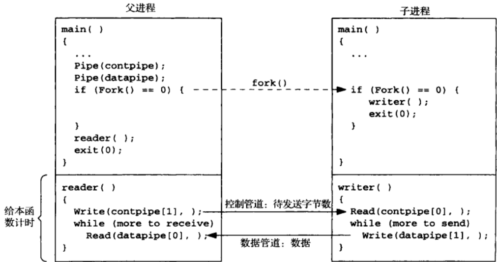
图A-14 测量一个管道的带宽的程序的概貌
