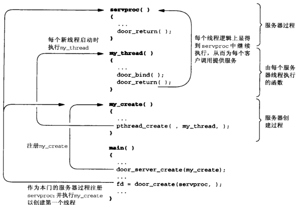
图15-21 我们的服务器进程中四个函数的概貌
