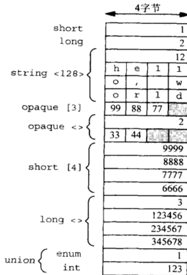
图16-20 由图16-18写出的XDR流的格式
