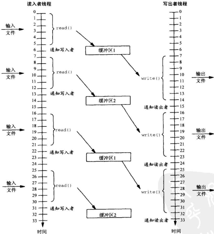
图10-32 双缓冲方案的时间线图
