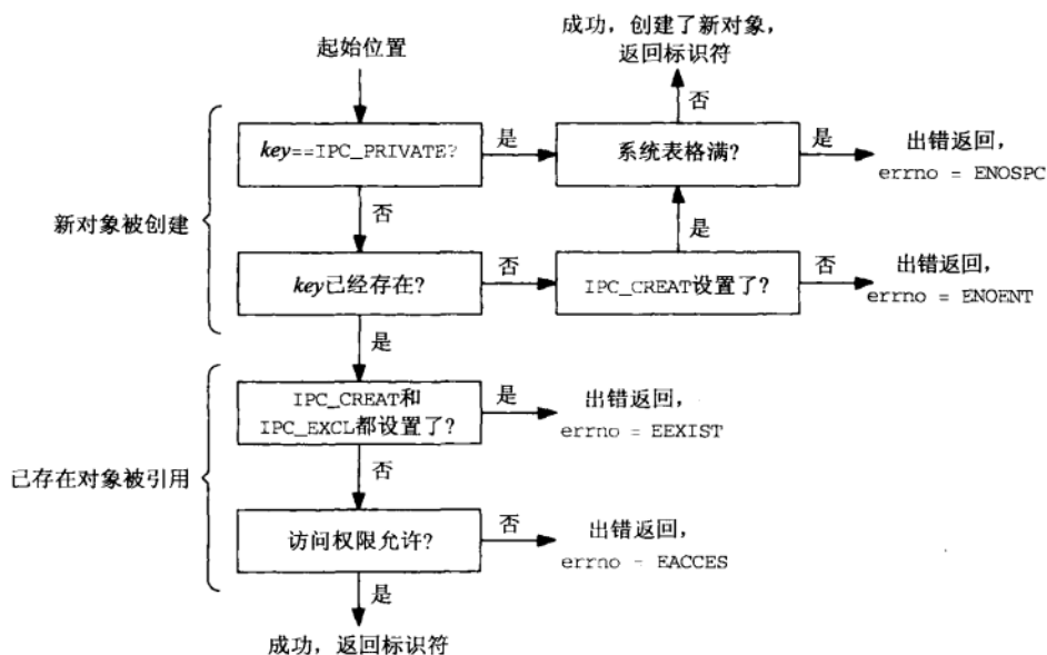
图3-4 创建或打开一个IPC对象的逻辑
