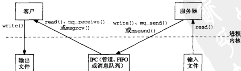
图12-1 从服务器到客户的文件数据流
