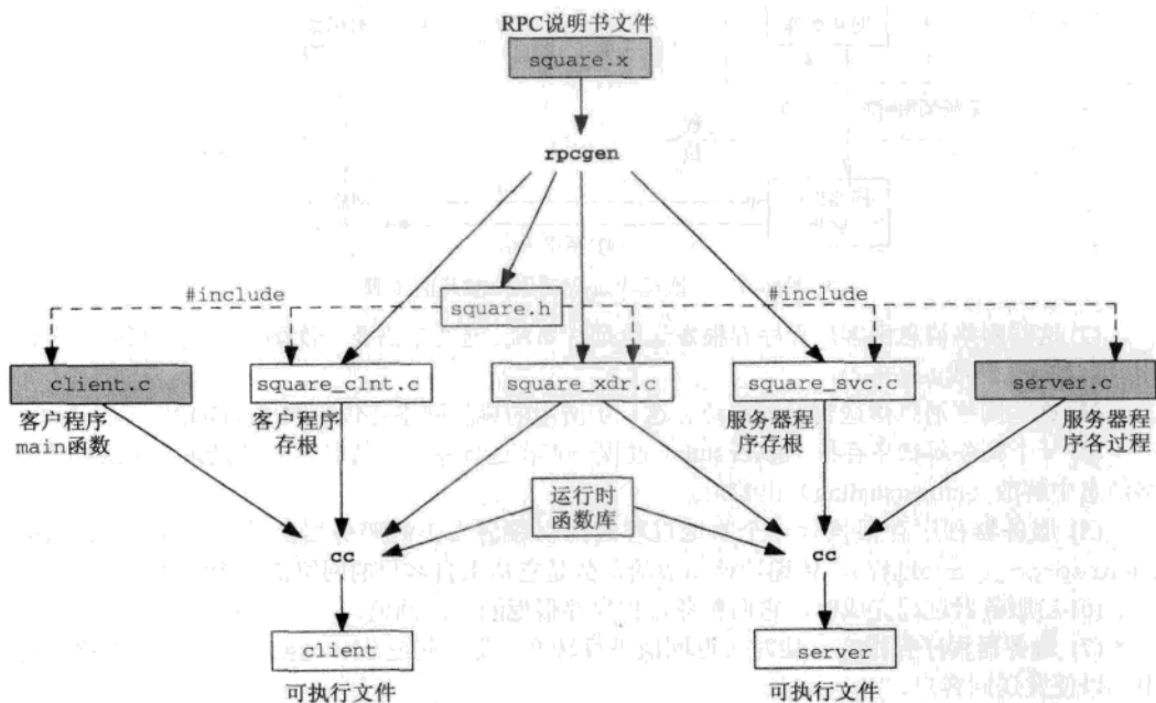
图16-4 构建一个RPC客户-服务器程序所需的步骤汇总
