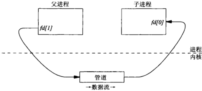
图4-4 两个进程间的管道
