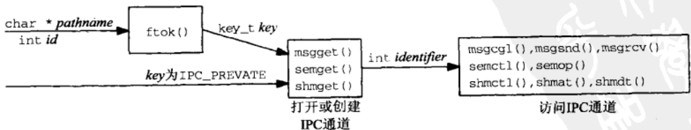
图3-3 从IPC键生成IPC标识符
