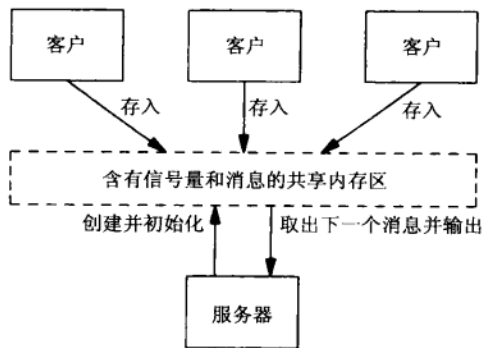
图13-9 多个客户通过共享内存区向一个服务器发送消息
