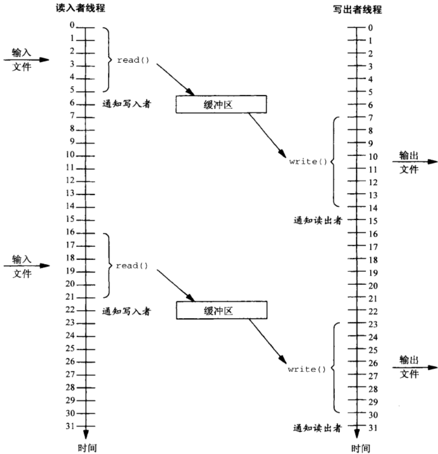
图10-30 把文件复制操作分割到两个线程中
