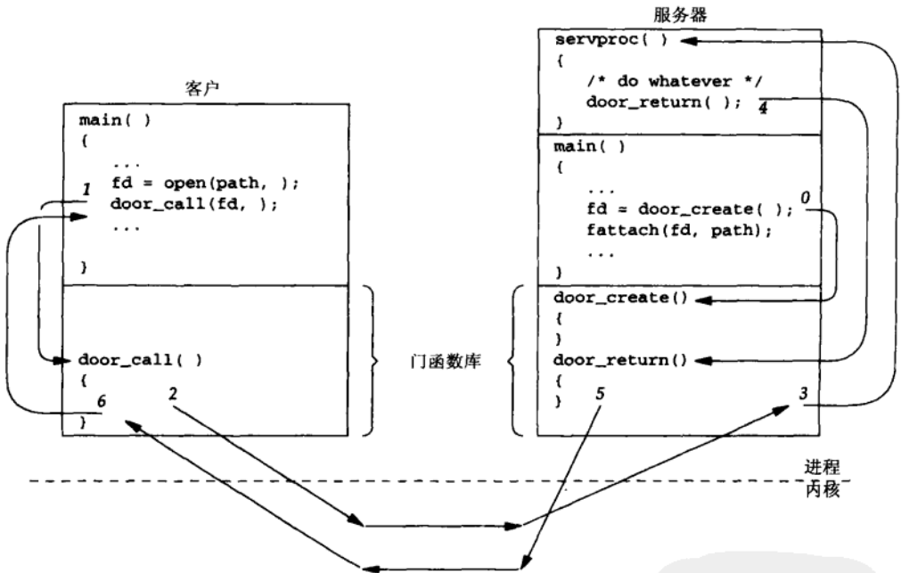
图15-5 从一个进程到另一个进程的过程调用的真正控制流
