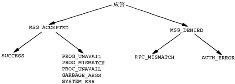
图16-31 可能的RPC应答
