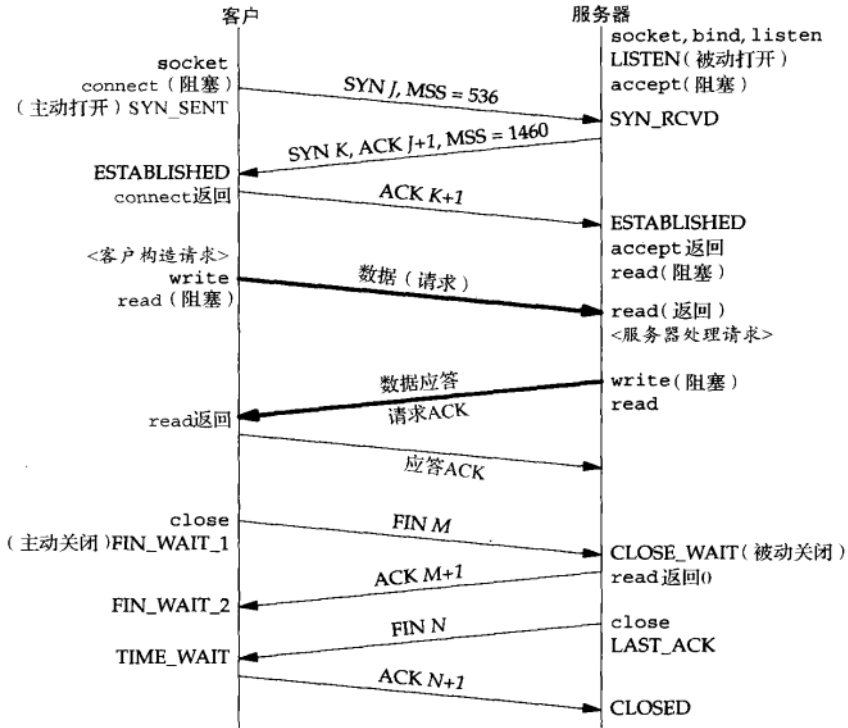
图2-5 TCP连接的分组交换
