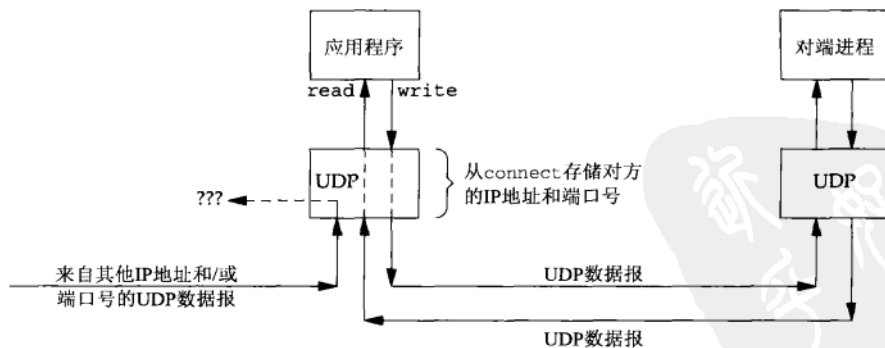
图8-15 已连接UDP套接字
