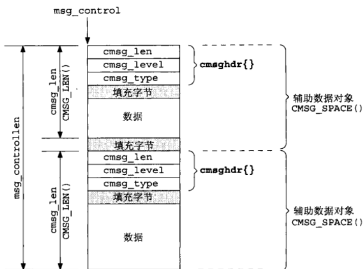
图14-12 包含两个辅助数据对象的辅助数据
