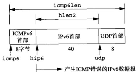
图28-22 处理ICMPv6错误涉及的首部、指针和长度
