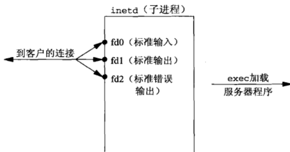
图13-10 dup2后子进程中的inetd描述符
