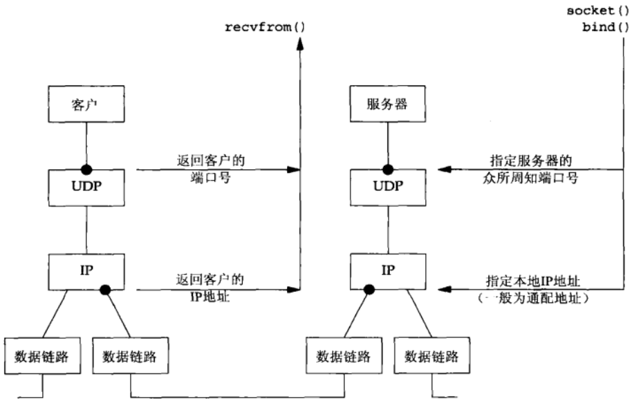
图8-12 从服务器角度总结UDP客户/服务器
