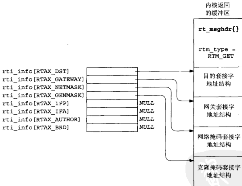
图18-8 get_rtaddrs函数填写的rti_info结构
