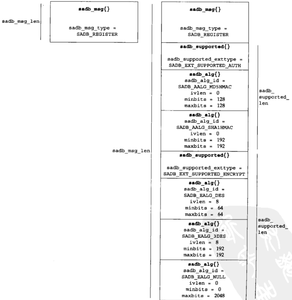
图19-14 内核为SADB_REGISTER请求返回的应答
