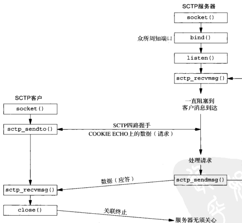
图9-2 SCTP一到多形式的套接字函数
