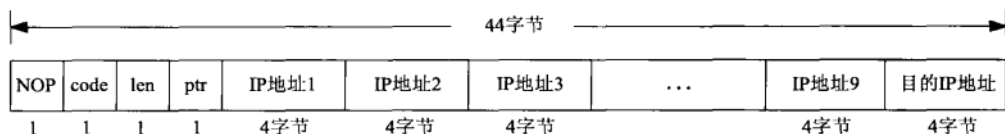
图27-1 向内核传递的源路径
