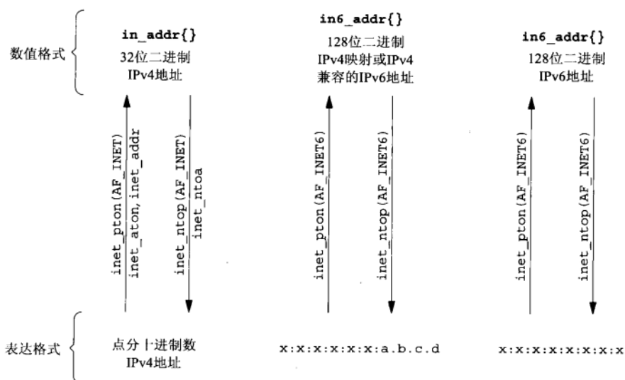
图3-11 地址转换函数小结
