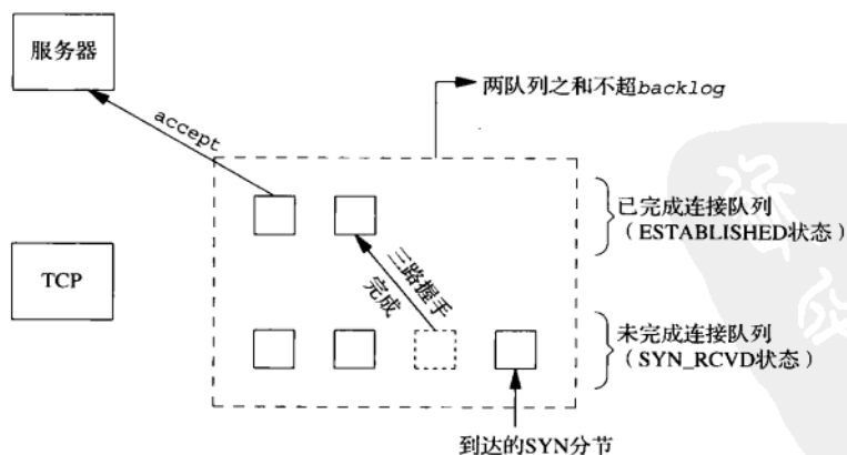
图4-7 TCP为监听套接字维护的两个队列
