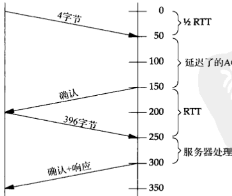
图E-6 Nagle算法与延滞ACK的交互情况
