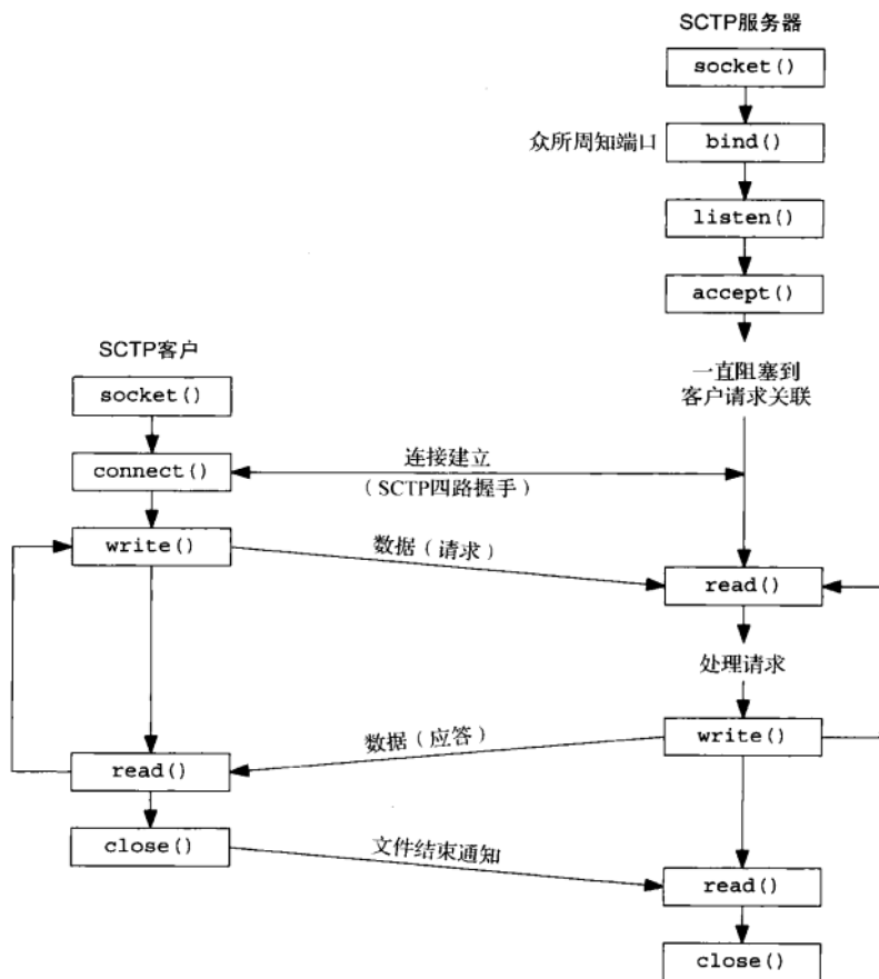
图9-1 SCTP一到一形式的套接字函数
