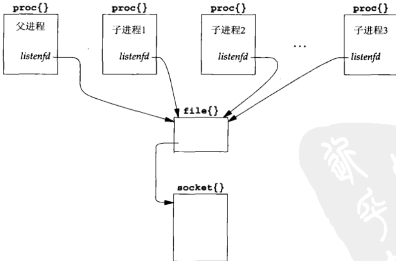
图30-13 proc、file和socket这三个结构之间的关系
