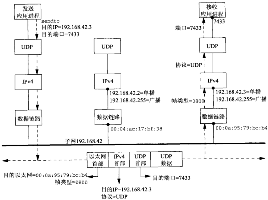
图20-3 UDP数据报单播示例
