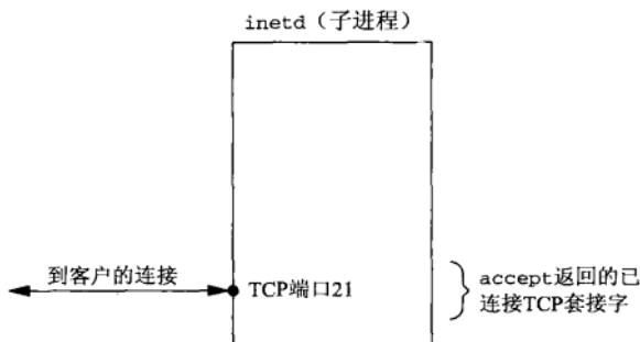
图13-9 子进程中的inetd描述符
