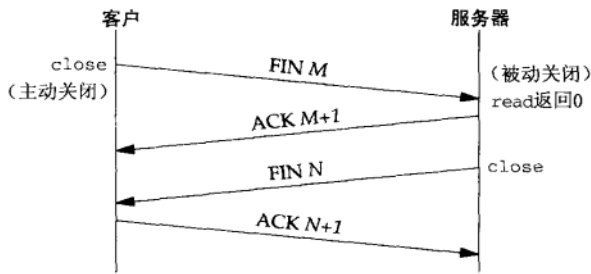
图2-3 TCP连接关闭时的分组交换
