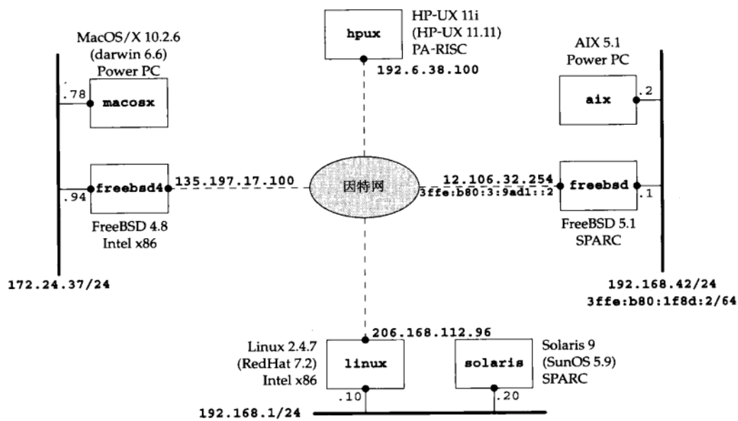
图1-16 本书示例所用的网络和主机
