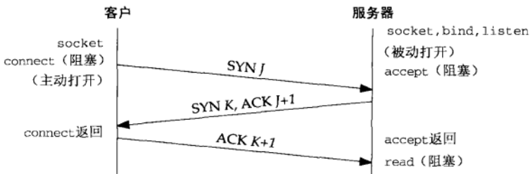
图2-2 TCP的三路握手
