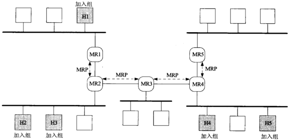
图21-6 广域网上5个主机加入一个多播组
