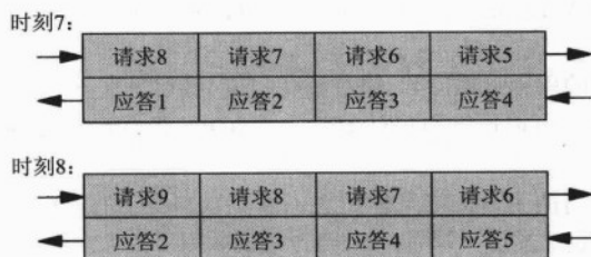
图6-11 填充客户与服务器之间的管道：批量方式
