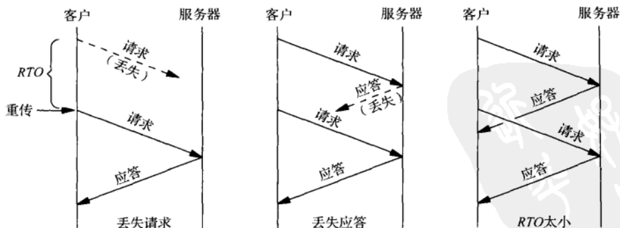
图22-5 重传定时器期满时的3种情形
