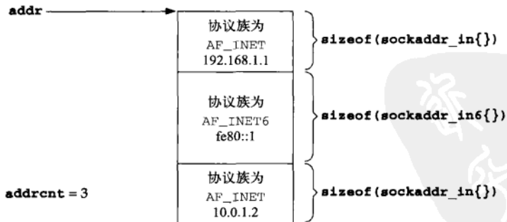
图9-4 SCTP调用所需的紧凑地址列表格式
