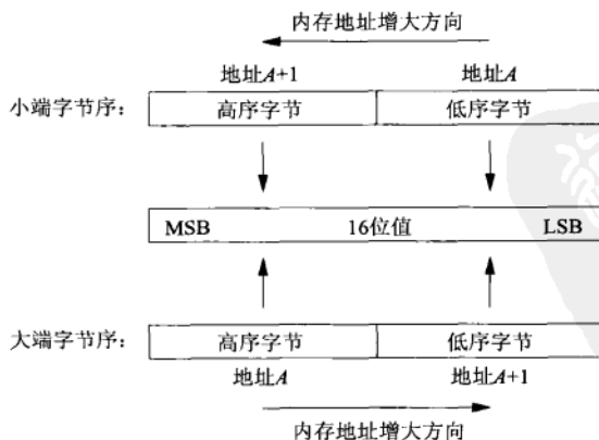
图3-9 16位整数的小端字节序和大端字节序
