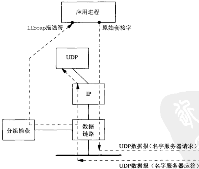
图29-3 检查某个名字服务器是否开启UDP校验和的应用程序
