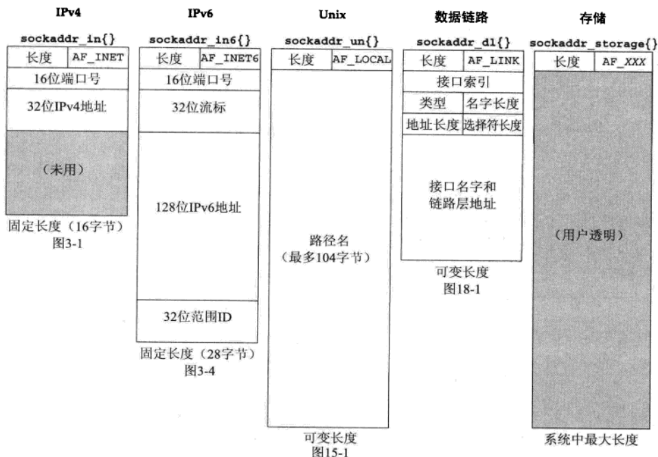
图3-6 不同套接字地址结构的比较
