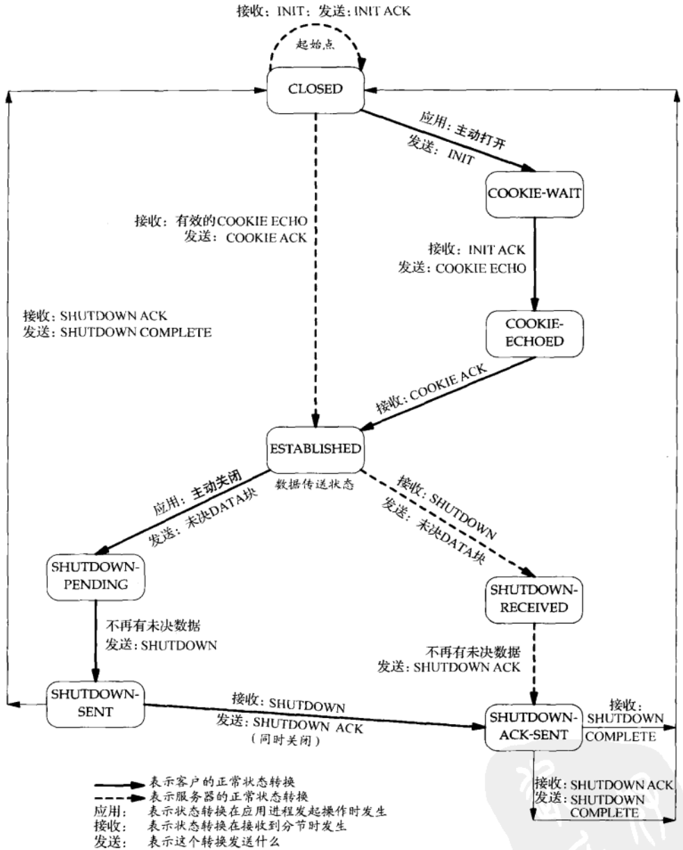
图2-8 SCTP状态转换图
