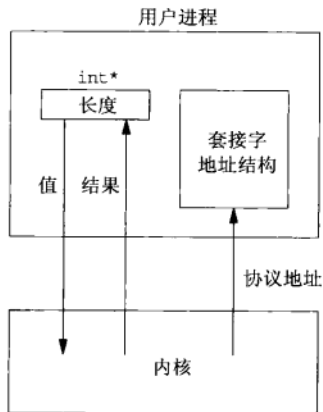
图3-8 从内核到进程传递套接字地址结构
