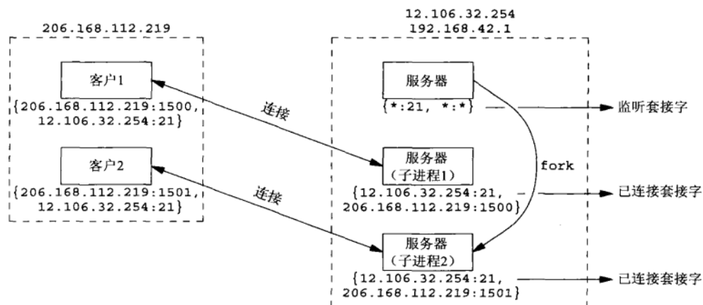
图2-14 第二个客户与同一个服务器的连接
