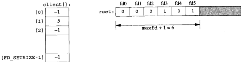
图6-20 第一个客户终止连接后的数据结构
