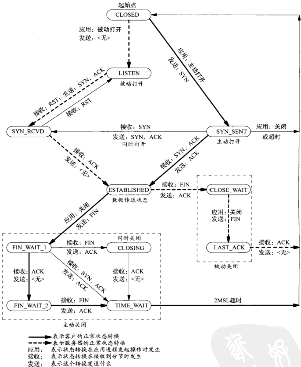
图2-4 TCP状态转换图
