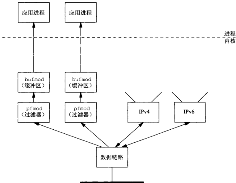
图29-2 使用DLPI、pfmod和bufmod捕获分组
