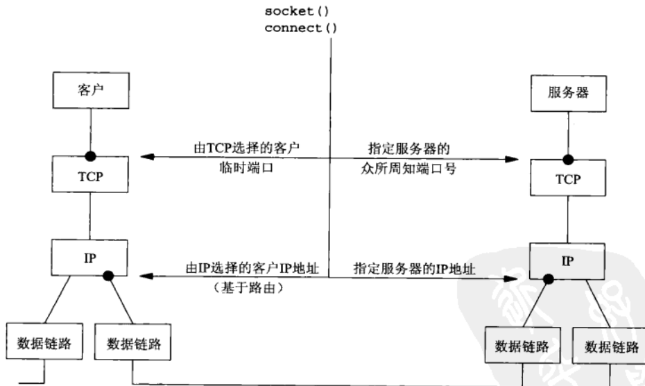
图5-15 从客户的角度总结TCP客户/服务器
