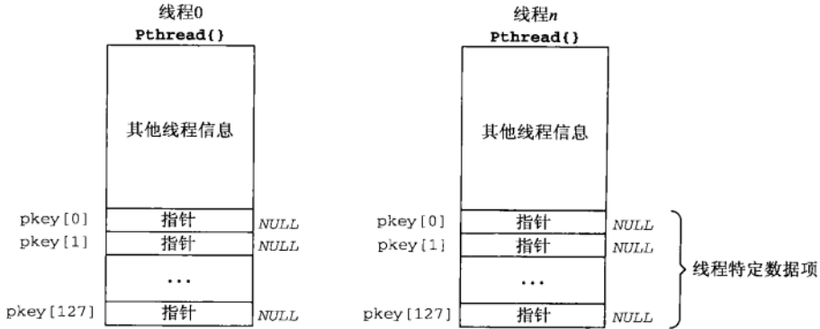
图26-8 系统维护的关于每个线程的信息
