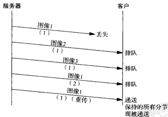
图10-5 在单个TCP连接上发送3幅图像
