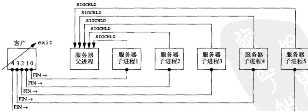
图5-10 客户终止，关闭5个连接，终止5个子进程
