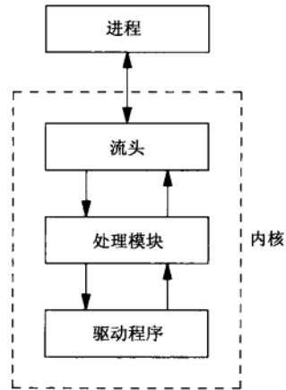
图31-2 压入一个处理模块的某个流
