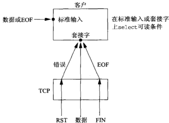
图6-8 str_cli函数中由select处理的各种条件
