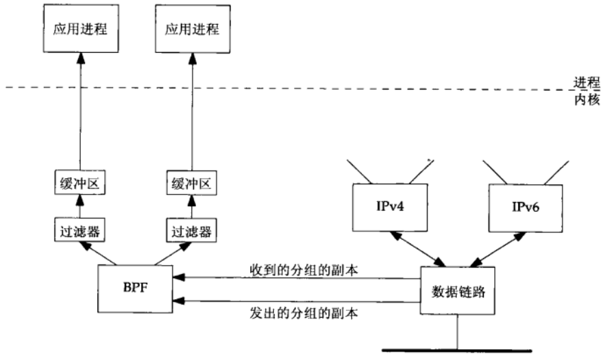
图29-1 使用BPF捕获分组
