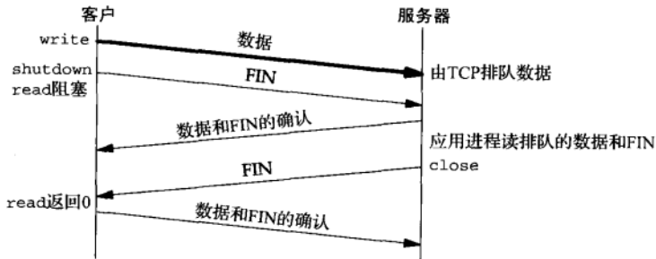
图7-10 用shutdown来获知对方已接收数据
