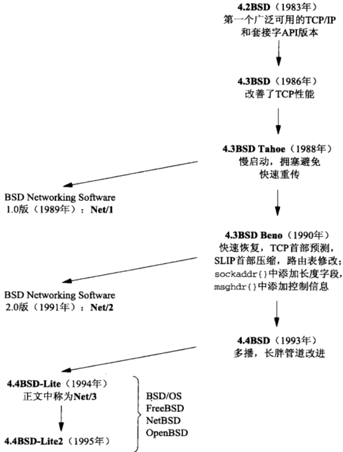
图1-15 各种BSD版本的历史
