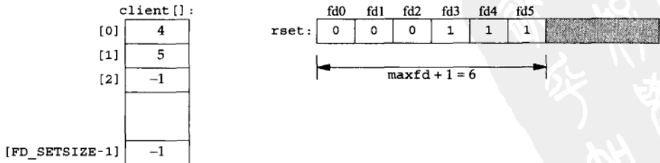
图6-19 第二个客户连接建立后的数据结构
