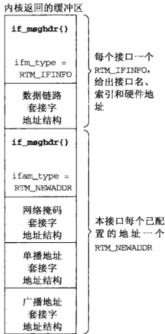
图18-13 由sysctl的CTL_NET/AF_ROUTE/NET_RT_IFLIST命令返回的信息
