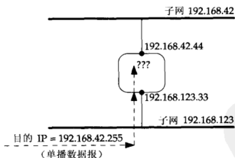
图20-2 路由器转发了网定向广播分组吗?
