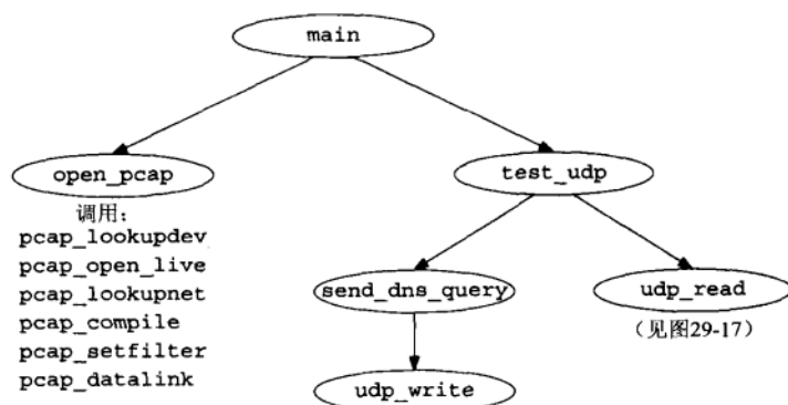
图29-4 udpcksum程序中的函数汇总
