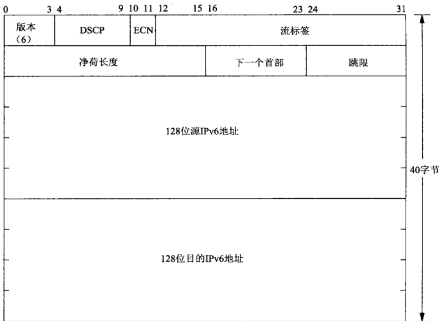
图A-2 IPv6首部格式
