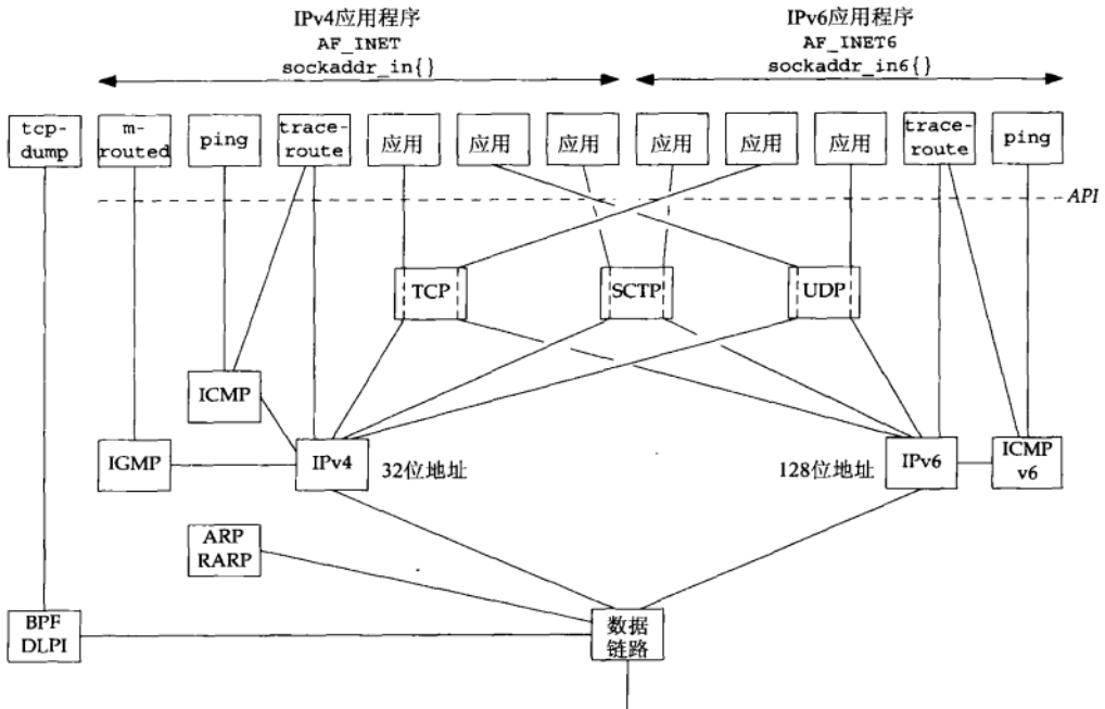
图2-1 TCP/IP协议概况
