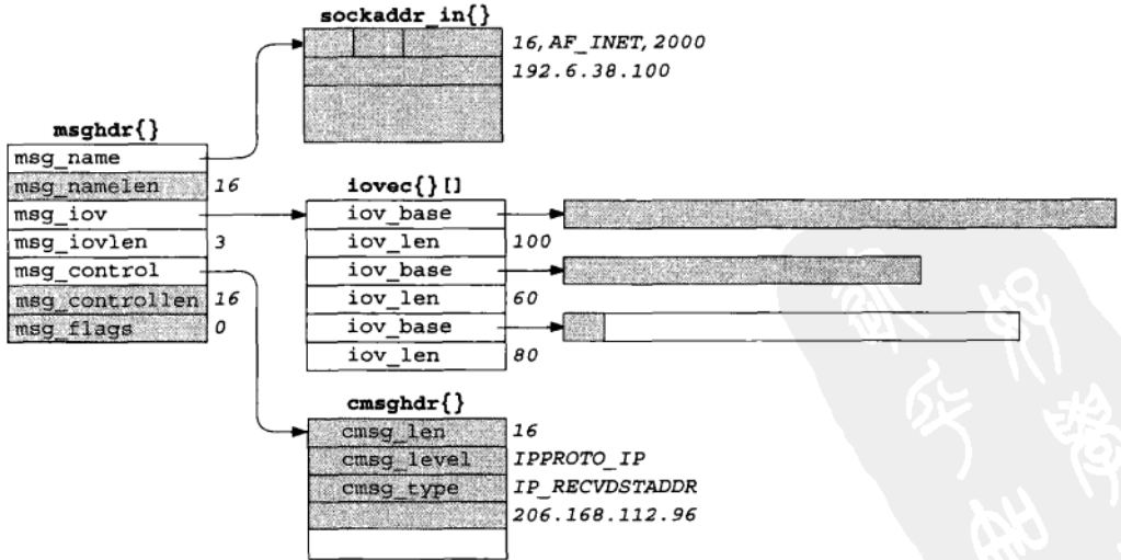
图14-9 recvmsg返回时对图14-8的更新
