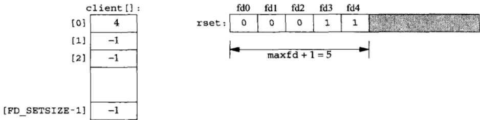
图6-17 第一个客户连接建立后的数据结构
