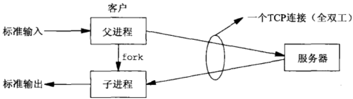
图16-9 使用两个进程的str_cli函数
