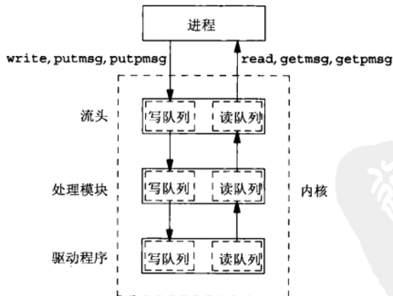
图31-4 流中每个部件至少有一对队列
