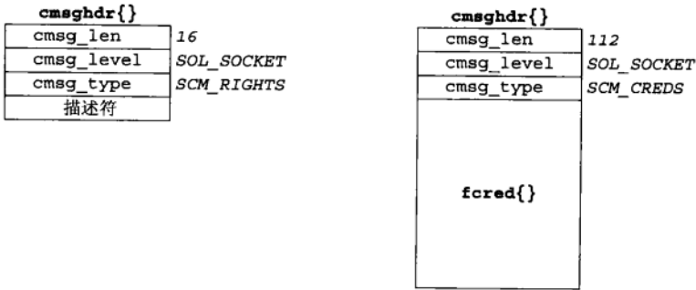
图14-13 用在Unix域套接字上的cmsghdr结构
