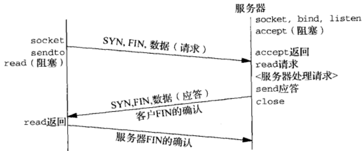
图14-19 最小T/TCP事务的时间线
