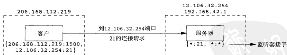
图2-12 客户对服务器的连接请求
