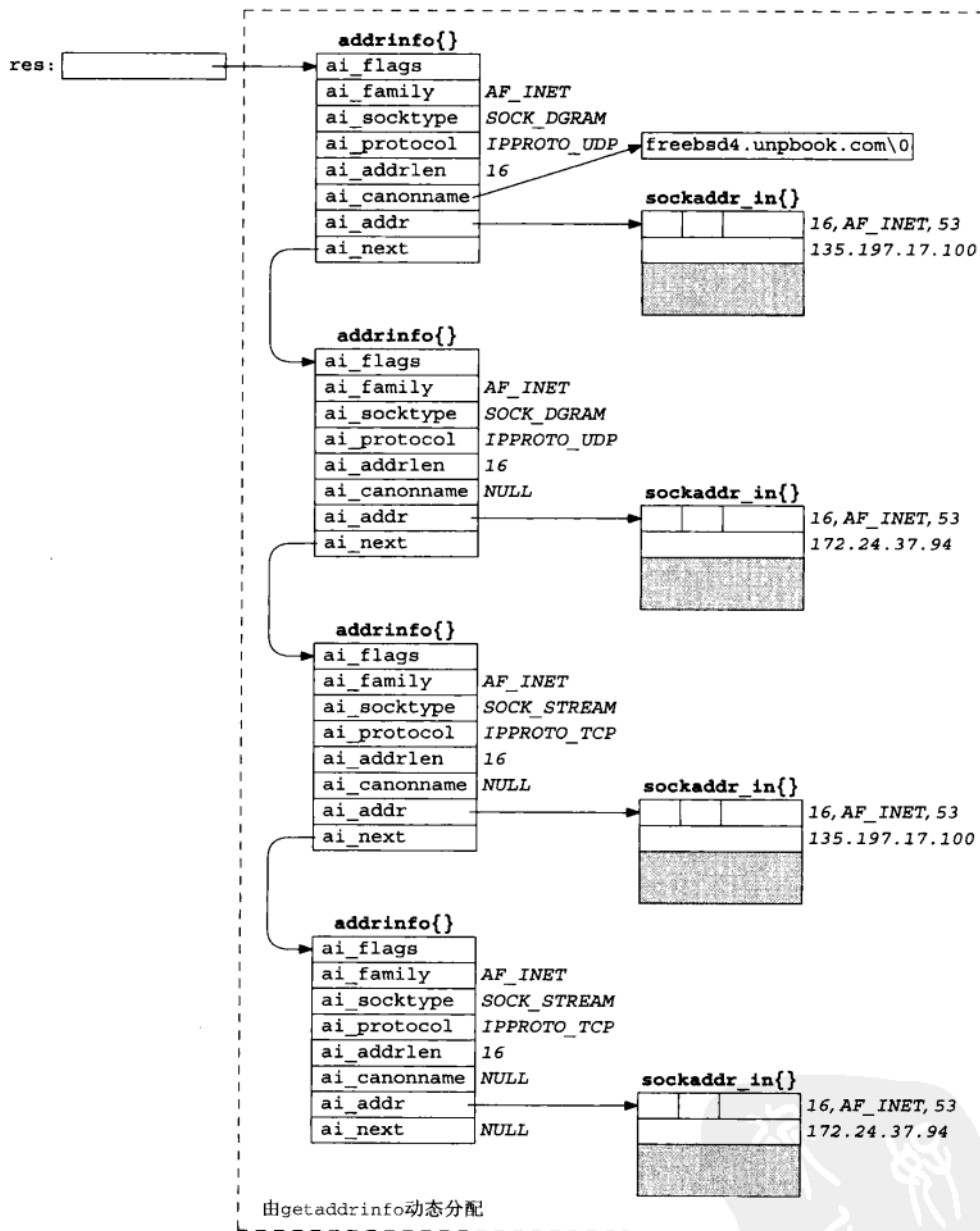
图11-5 getaddrinfo 返回信息的实例
