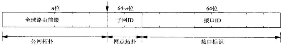
图A-8 IPv6全球单播地址一般格式
