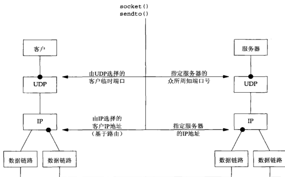
图8-11 从客户角度总结UDP客户/服务器
