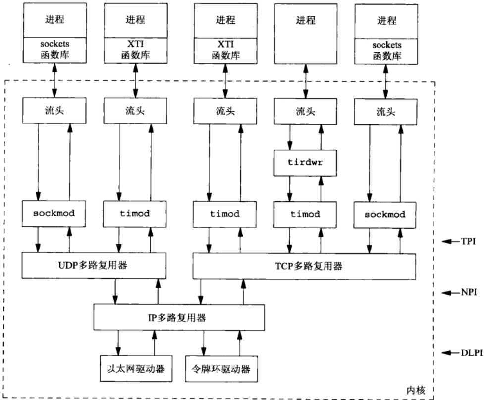
图31-3 TCP/IP基于流的某种可能的实现
