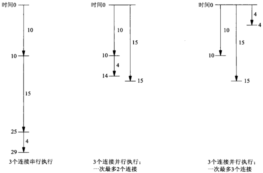
图16-12 并行建立多个连接
