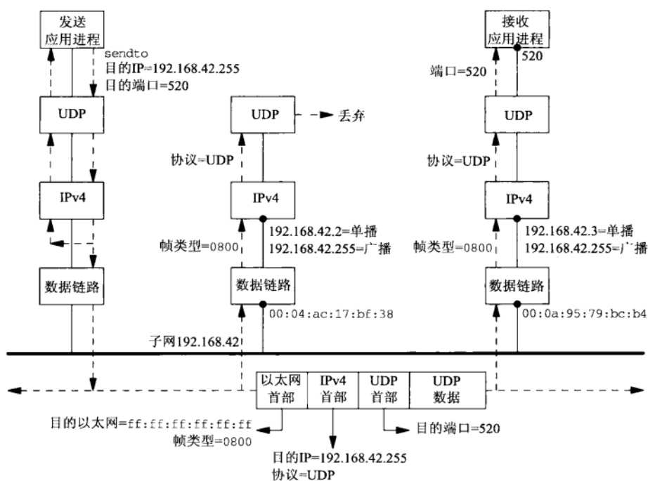
图20-4 UDP数据报广播示例
