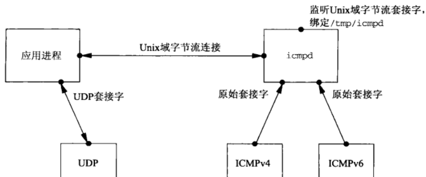
图28-27 应用进程创建自身的UDP套接字和到 icmpd 的Unix域连接
