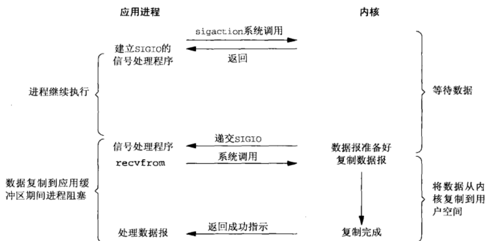
图6-4 信号驱动式I/O模型
