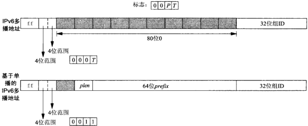
图21-2 IPv6多播地址格式
