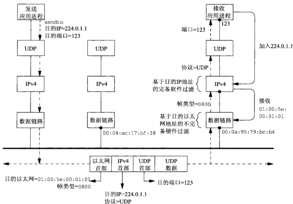
图21-4 UDP数据报多播示例
