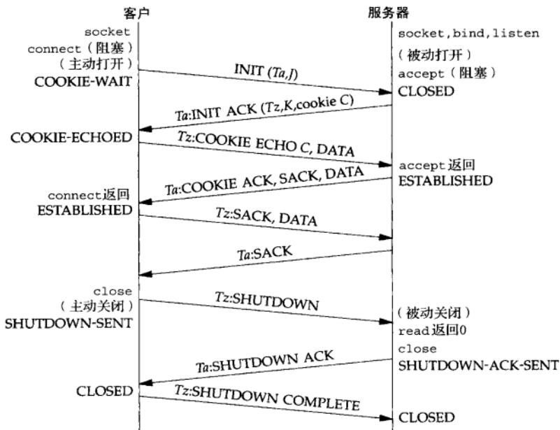
图2-9 SCTP关联中的分组交换
