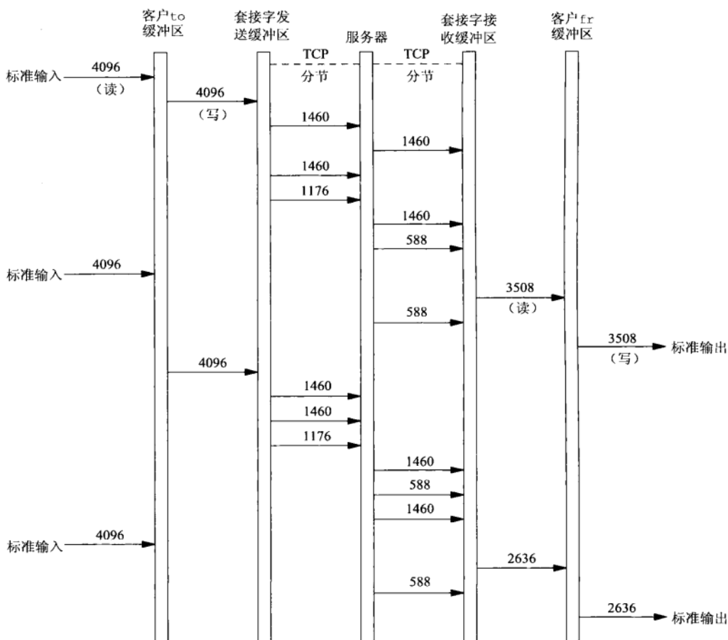
图16-8 非阻塞式I/O例子的时间线
