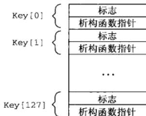
图26-7 线程特定数据的可能实现
