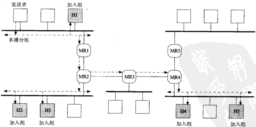
图21-7 广域网上发送多播分组
