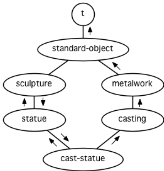
图 11.3: 类别层级
