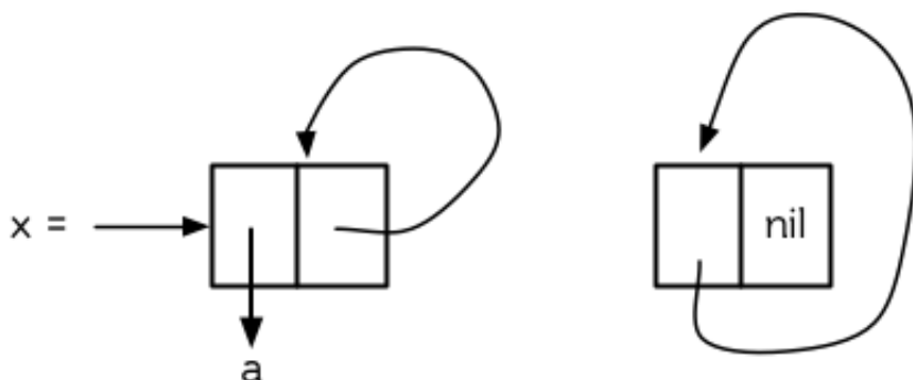
图 12.12 环状列表。
