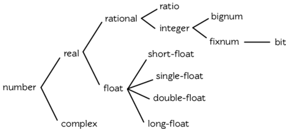
图 9.1: 数值类型
