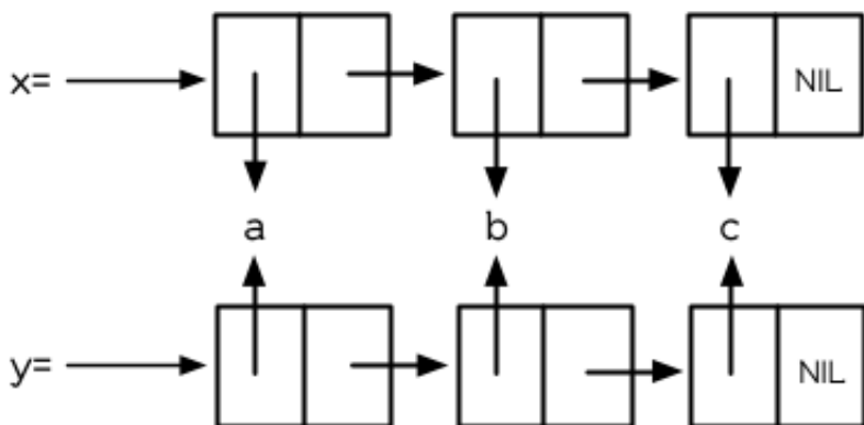
图 3.5 复制的结果
