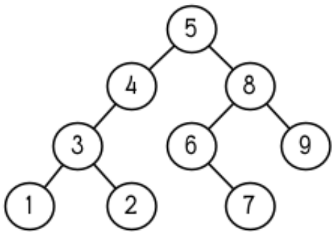
图 4.4: 二叉搜索树
