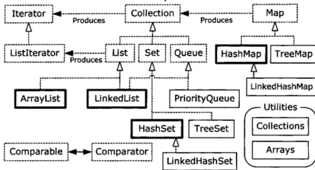
简单的容器分类
