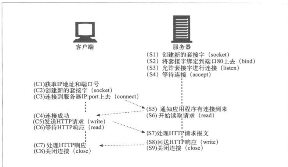
图 4-6 TCP 客户端和服务器的如何通过 TCP 套接字接口进行通信的
