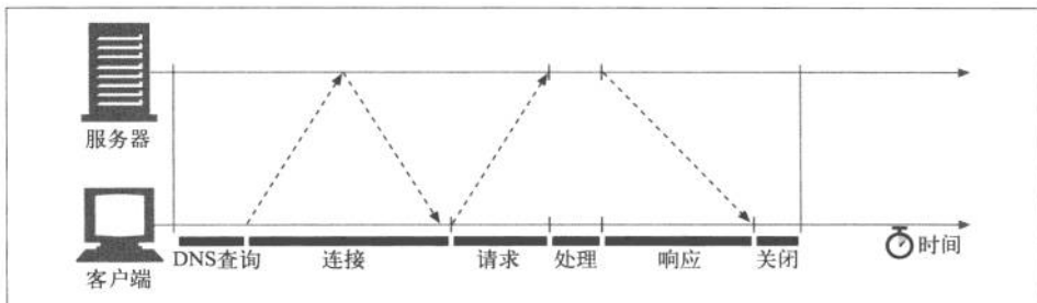
80 图 4-7 串行 HTTP 事务的时间线
