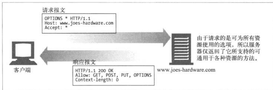
图 3-12 OPTIONS 示例
