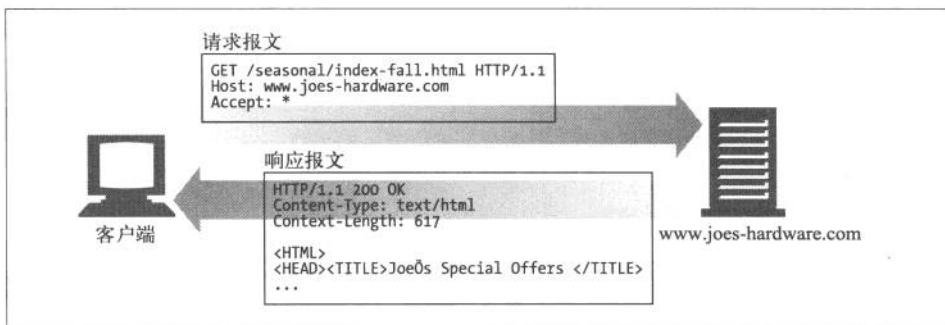
图 3-7 GET 示例
