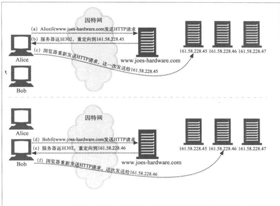
图 20-1 HTTP 重定向
