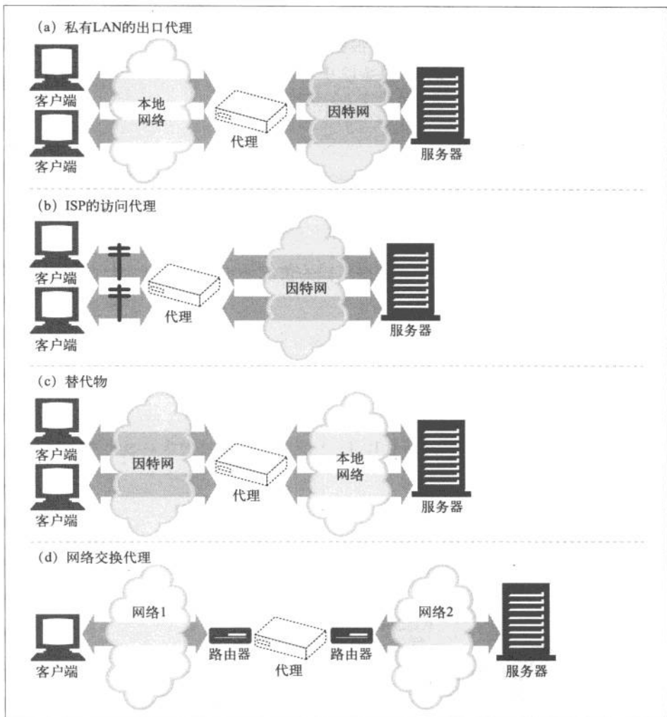
图 6-11 可以根据其目标用途，以多种方式来部署代理
