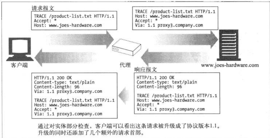
图 3-11 TRACE 示例
