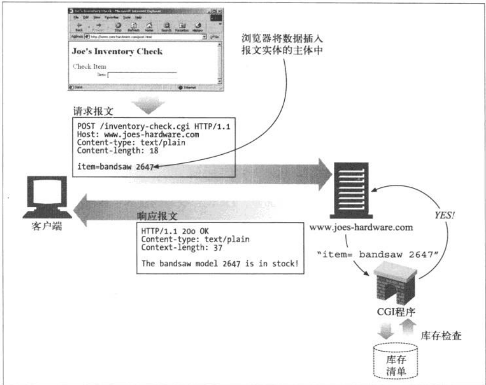
图 3-10 POST 示例
