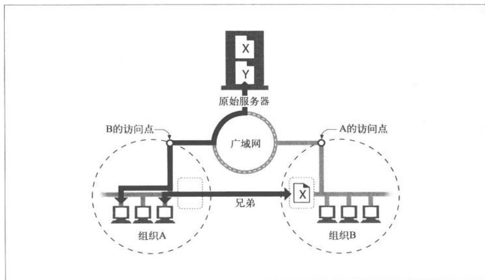
图 7-10 兄弟缓存
