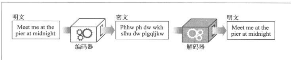
图 14-3 明文和密文
