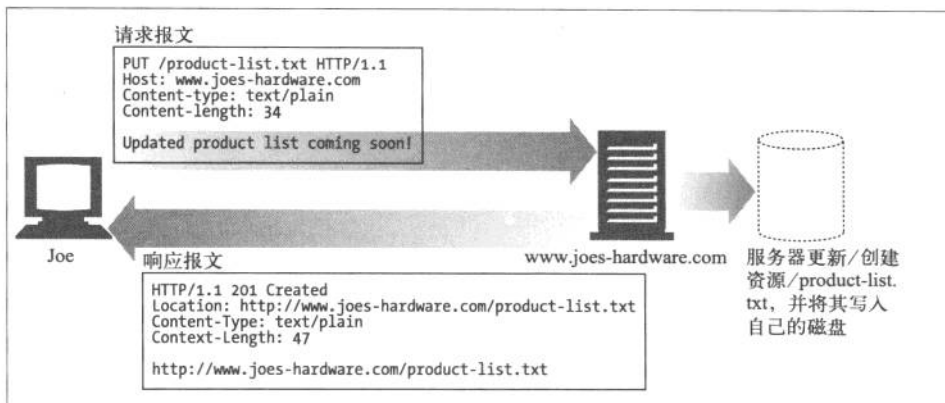
图 3-9 PUT 示例
