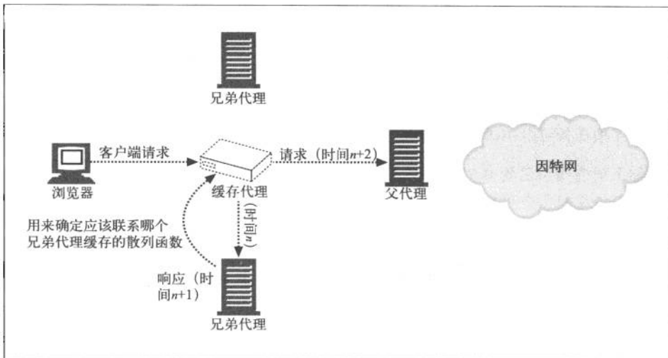
图 20-14 CARP 重定向
