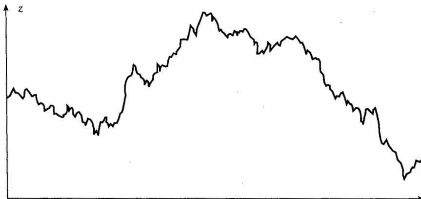
图 12-1 当式(12-1)中 \Delta t \rightarrow 0 时, 维纳过程的产生方式
