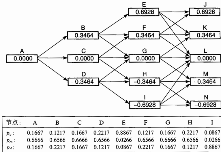
图 33-1 X 的树形
