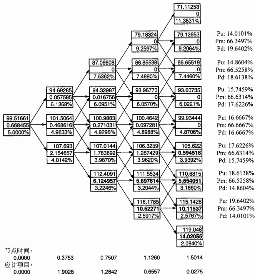
图 30-11 对美式债券期权定价的树形，该图由 DerivaGem 软件生成
