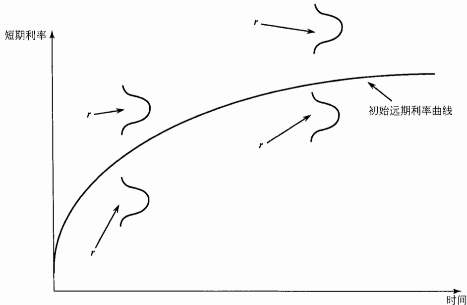
图 30-4 Hull-White 模型
