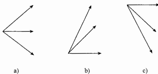
图 30-7 三叉数中的不同树枝形状
