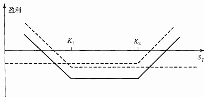
图 10-12 异价跨式期权的收益
