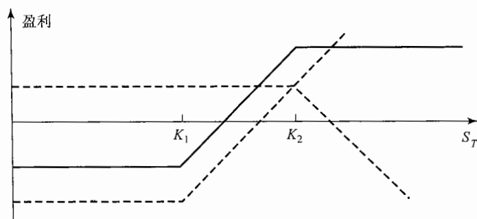
图 10-2 由看涨期权所构造的牛市差价的盈利
