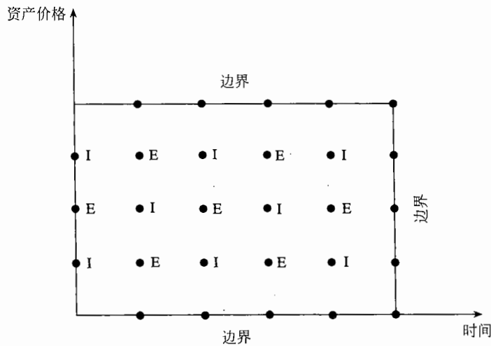
图 19-18 跳格差分法
