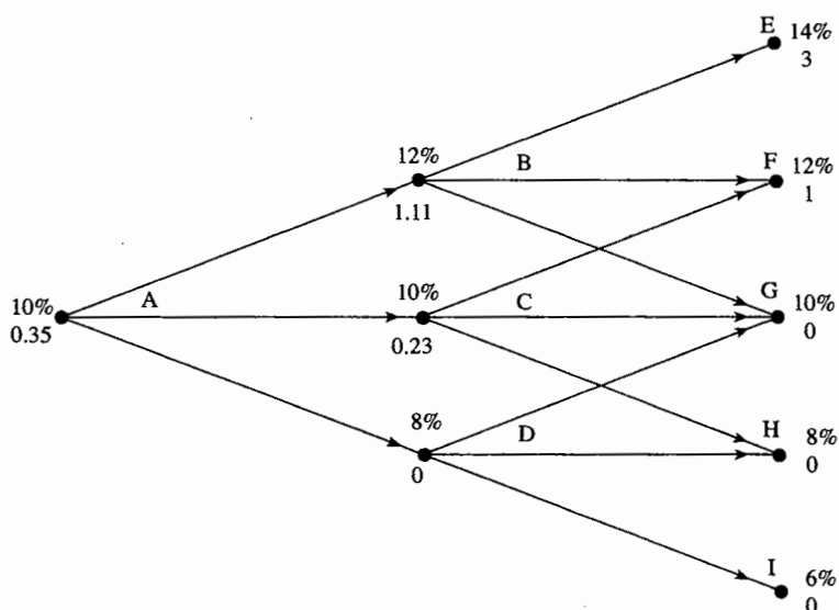
图 30-6 三叉树应用实例
