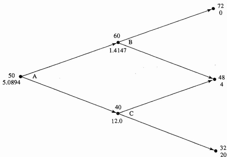
图 11-8 利用两步二叉树来对美式看跌期权定价
