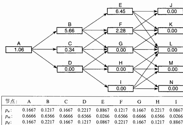
图 33-5 对含有扩大期权的项目进行评估
