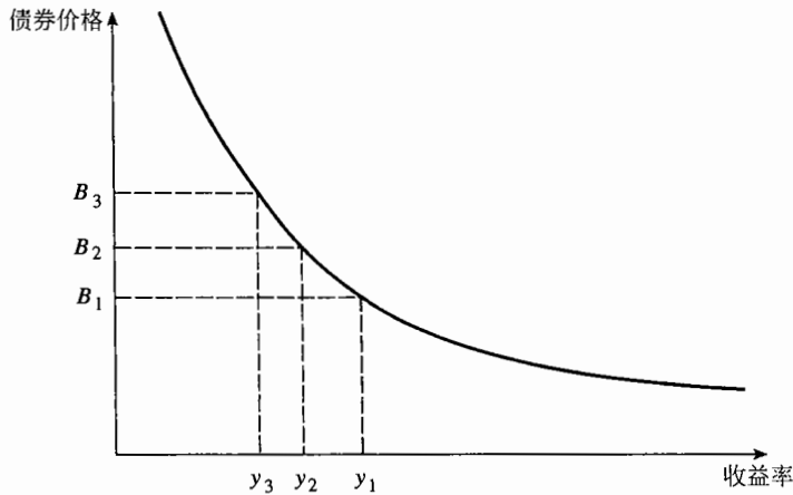
图 29-1 在时间 T 时债券价格与债券收益率的关系
