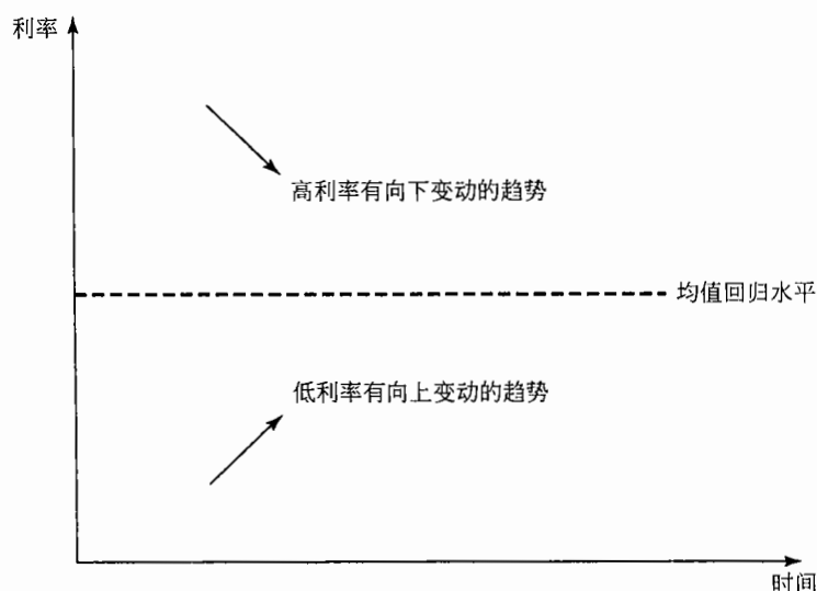
图 30-1 均值回归
