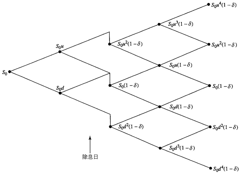
图 19-7 当在某指定时刻支付一定股息收益率的股票的二叉树
