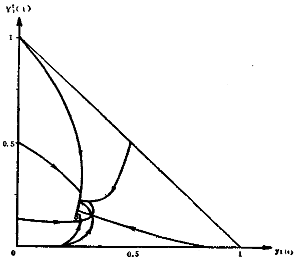
图A-2 (y_1, y_3^t) 相位平面上的典型轨迹
