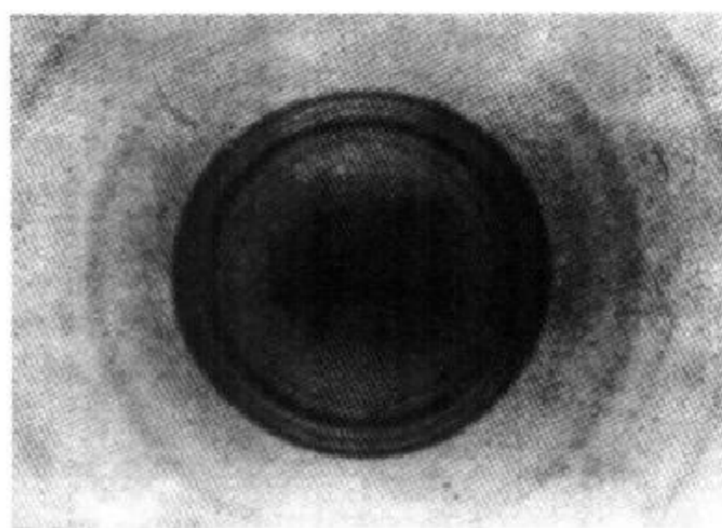
附图IV X射线的衍射 (Lastowiecki 及 Gregor 摄)
