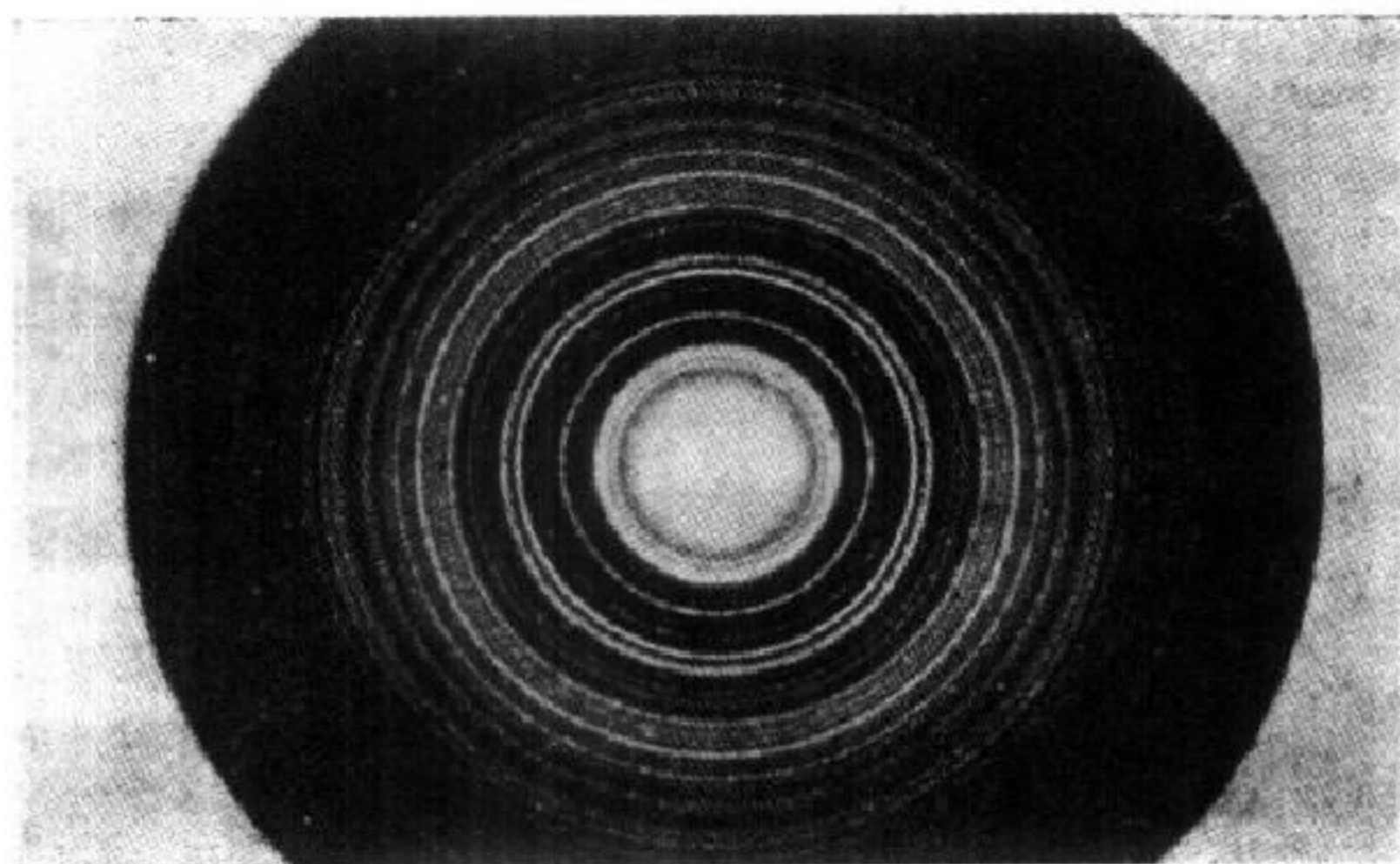
附图V 电子波的衍射 (Loria 及 Klinger 摄)
