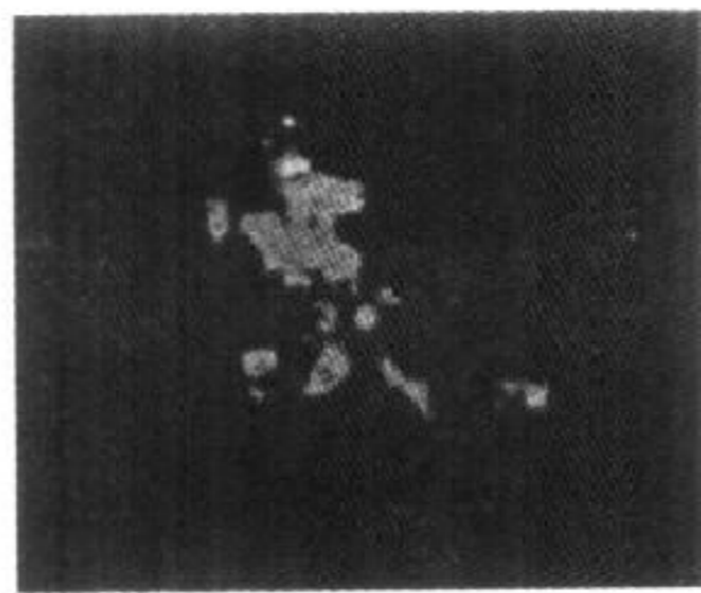
附图 1b 用慢镜头拍摄下来的一个布朗粒子 (Brumberg 及 Vavilov 摄)
