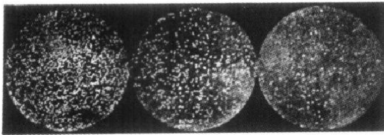
附图 1a 显微镜中看到的布朗粒子 (F. Perrin 摄)
