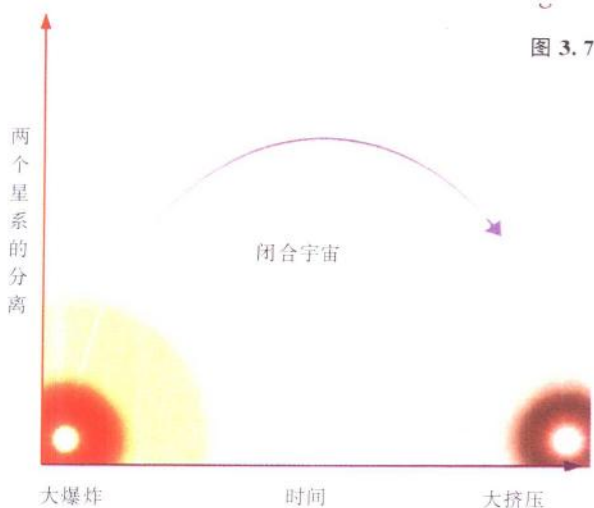
图 3.7 在弗利德曼的宇宙模型中所有星系一开始都相互离开。宇宙一直膨胀到它的最大尺度，然而被收缩回到—点
