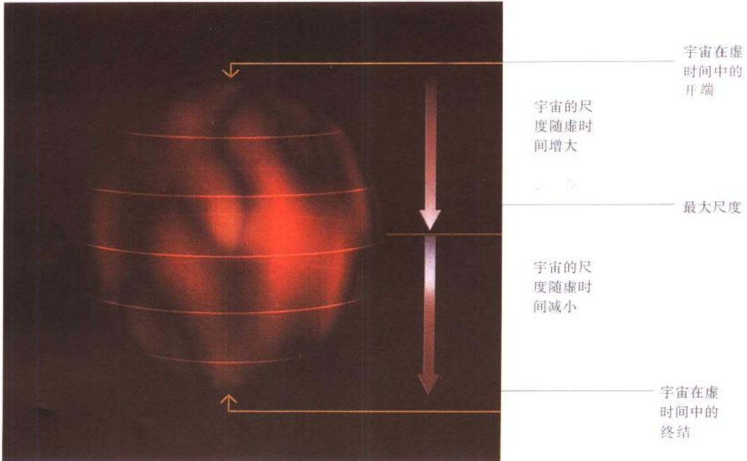
宇宙
