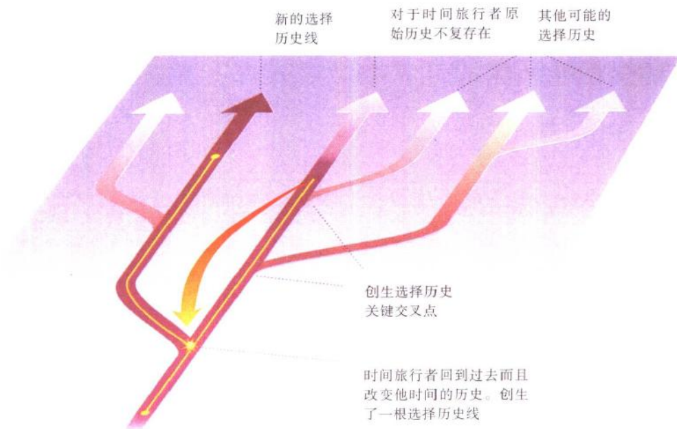
图 10.9 解决时间旅行佯谬的一种方法是假定存在选择历史整个系列,它们在某些关键事件处相互分叉。
