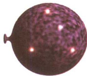
膨胀气球理论
