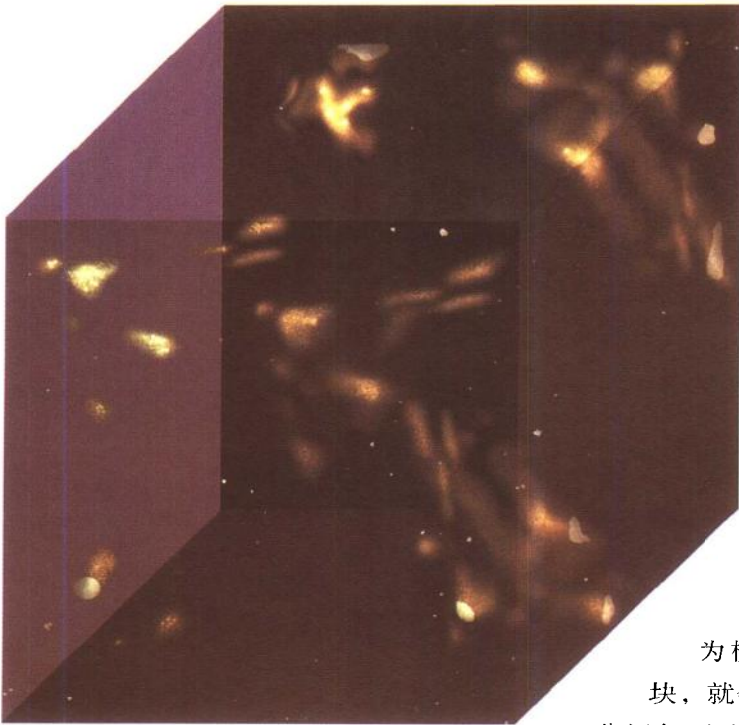
星系团
