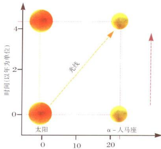
离开太阳的距离(以 10^{12} 英里为单位)
