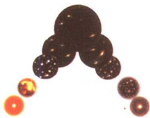
弗利德曼闭合宇宙
