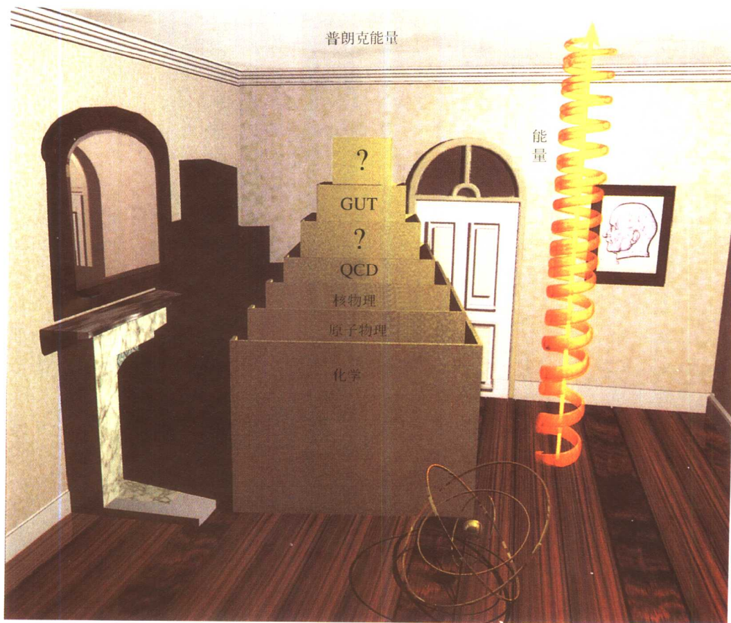
图 11.16 对越来越小尺度的观测导致直至量子色动力学(QCD)的在越来越高能量下成立的物理理论序列,甚至可能还要超过直至大统一理论(GUT)。然而,普朗克能量可以提供一个切断,并且暗示存在的一个终极理论。
