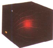
历史求和模型
