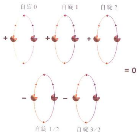
图 11.4 自旋 1/2 和 3/2 的虚对的能量是负的，并把自旋 0, 1 和 2 的对的正能量抵消，这就排除了大多数的无穷大。
