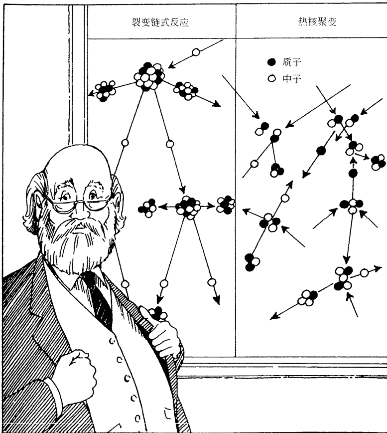
聚变和裂变都能够释放出能量
