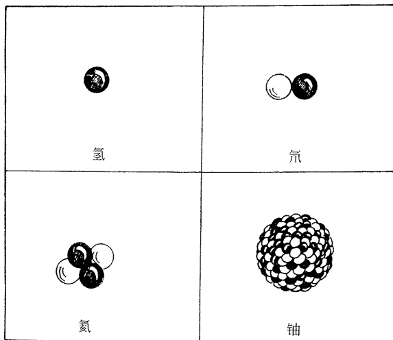
氢、氦、锂和铀的原子核
