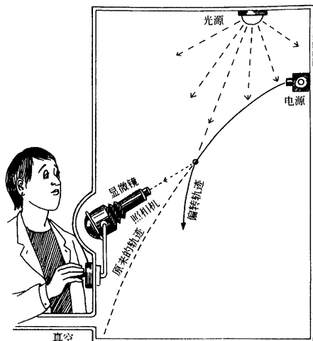
光可能干扰物体的运动
