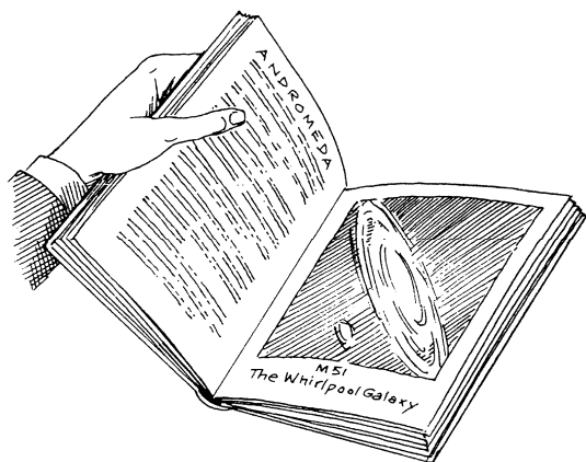
你可以在各种天文学书籍中找到仙女座的照片
