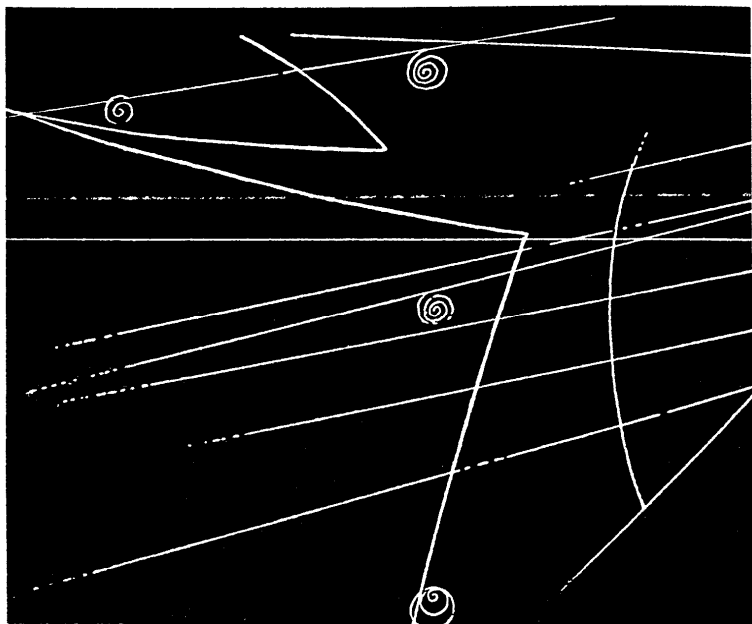
一个成对产生的事件
