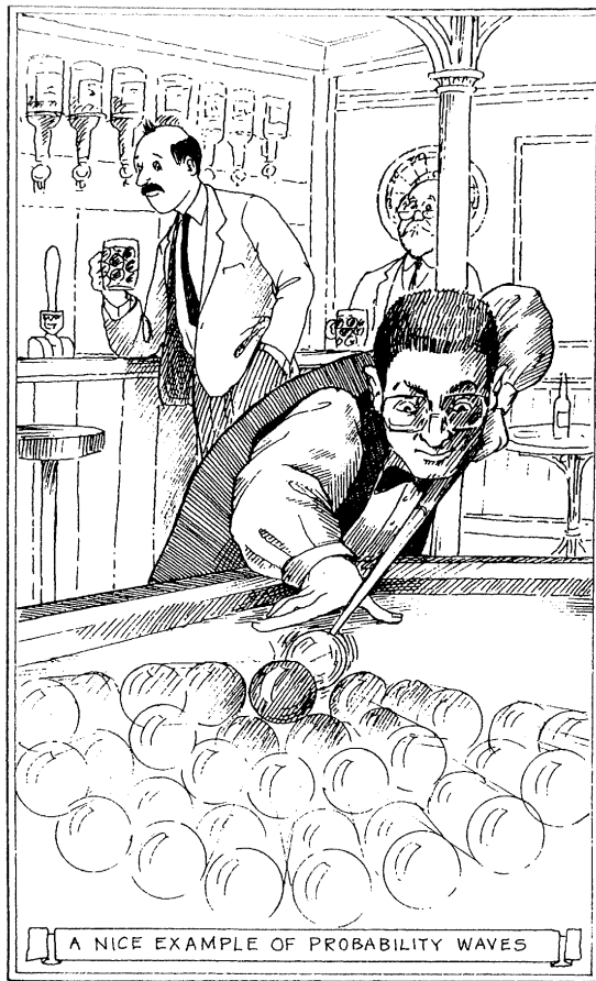
这是概率波的一个很好的事例
