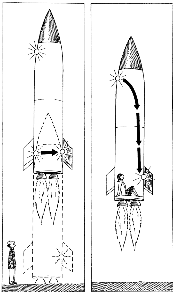
穿过加速飞行的飞船的光线
