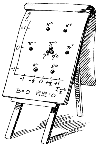
同样完整的六角形
