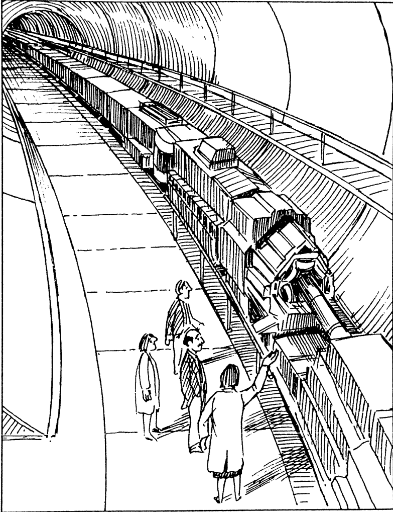
粒子在这种管道内运动
