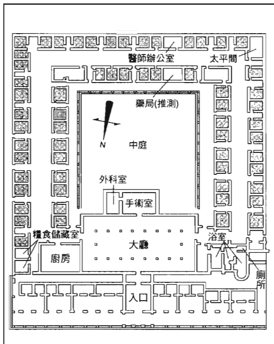
占田軍團基地中軍醫院的平面圖(■的房間為病房)
