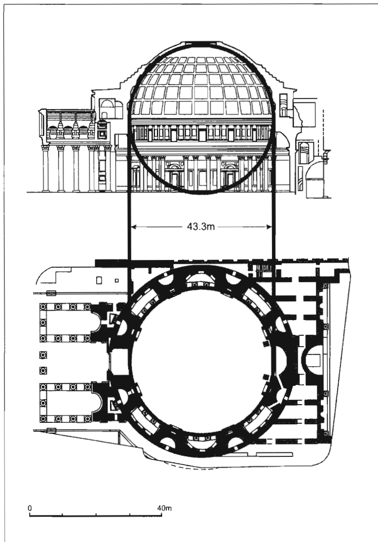
萬神殿（斷面圖與平面圖）
