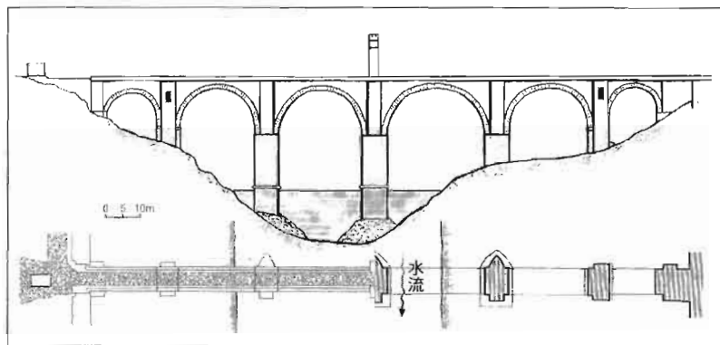
橋樑的側面圖(上)與平面圖(下)
