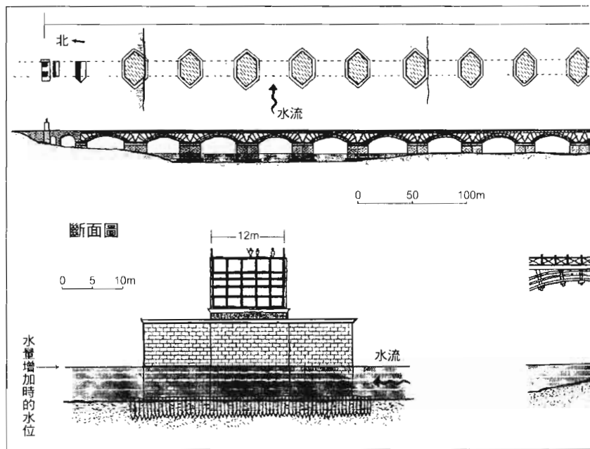
圖拉真橋（復原圖。最上段是由上往下看的橋身平面圖）
