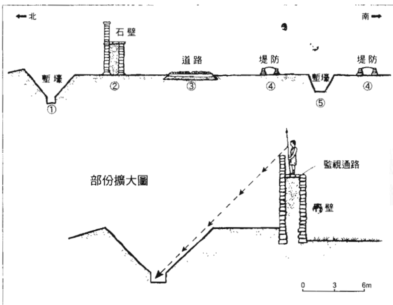
石壁部份（沒有塔、城塞等的段落）的斷面圖
