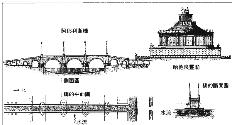
哈德良靈廟與阿耶利斯橋（復原圖）
