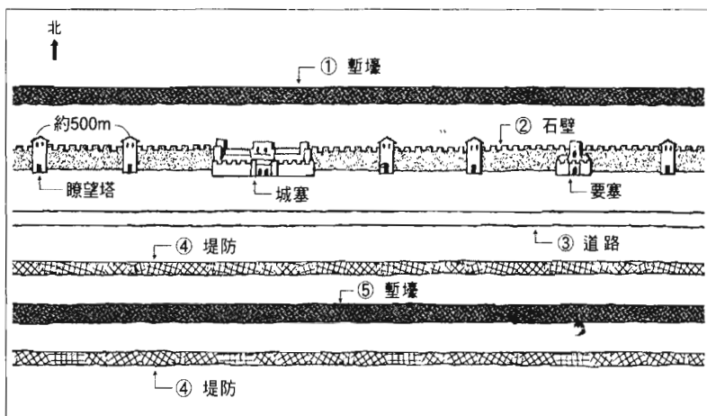
「哈德良長城」模型圖
