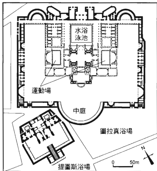
比鄰而立的二皇帝的浴場
