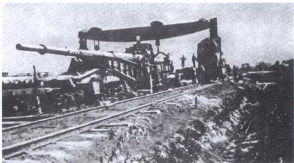
■ 如果要評選第一次世界大戰中最有「傳奇性武器」味道的一種秘密武器，我想這項榮譽一定非「巴黎大砲」莫屬。由於身管超長，在配合的大量發射藥之後，彈丸在飛出砲體的瞬間能達到極高的速度，大仰角射擊又使其可以向上一直飛入同溫層，最後在劃出一個巨大的弧線之後落入100多公里之外的目標——巴黎。右圖為巴黎大砲進入發射陣地前的運輸狀態，這個大傢伙的就位和發射可不是簡單的工作。
