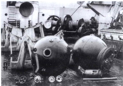
■ 德軍佈雷艦上的水雷。
